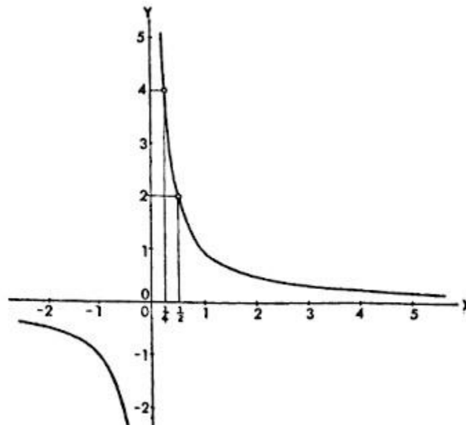
Figura 128. Gráfica de la función y = 1/x
