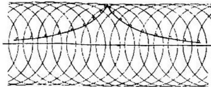
Figura 45(b). La tractriz también es la curva que es perpendicular a
