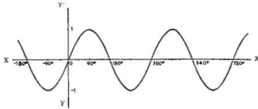
Figura 22(b). Representación gráfica de la ecuación y = \text{sen } x . Ésta es la famosa curva ondulada que se emplea para representar muchos fenómenos periódicos y regulares, por ejemplo, la corriente eléctrica, el movimiento de un péndulo, la radio transmisión, las ondas sonoras y luminosas, etc. (Para el significado de \text{sen } x , véase la nota 2 en el capítulo sobre el cálculo infinitesimal.)
