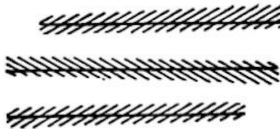
Figura 71. ¿Son paralelas las tres rectas horizontales?
