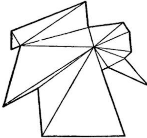
Figura 137. Se determina la superficie de este polígono irregular, formando los triángulos indicados y calculando el área de cada uno de ellos.
