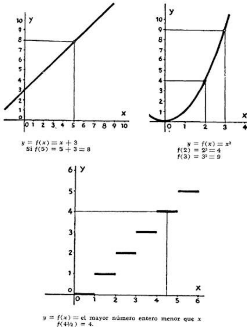
Figura 127. Representaciones de tres funciones diferentes.
