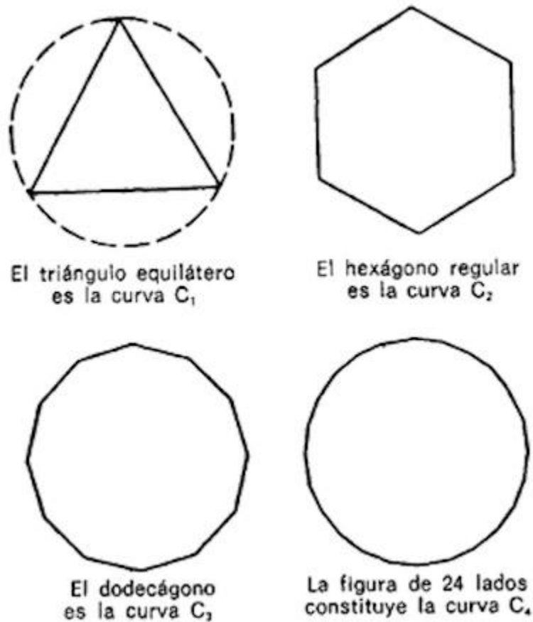
Figuras. 141, 142, 143, 144. El círculo considerado como curva límite de una sucesión de curvas.
