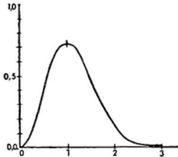
Figura 81. Velocidad de las moléculas de un gas.
