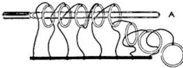
Figura 52. El rompecabezas de los anillos chinos.
