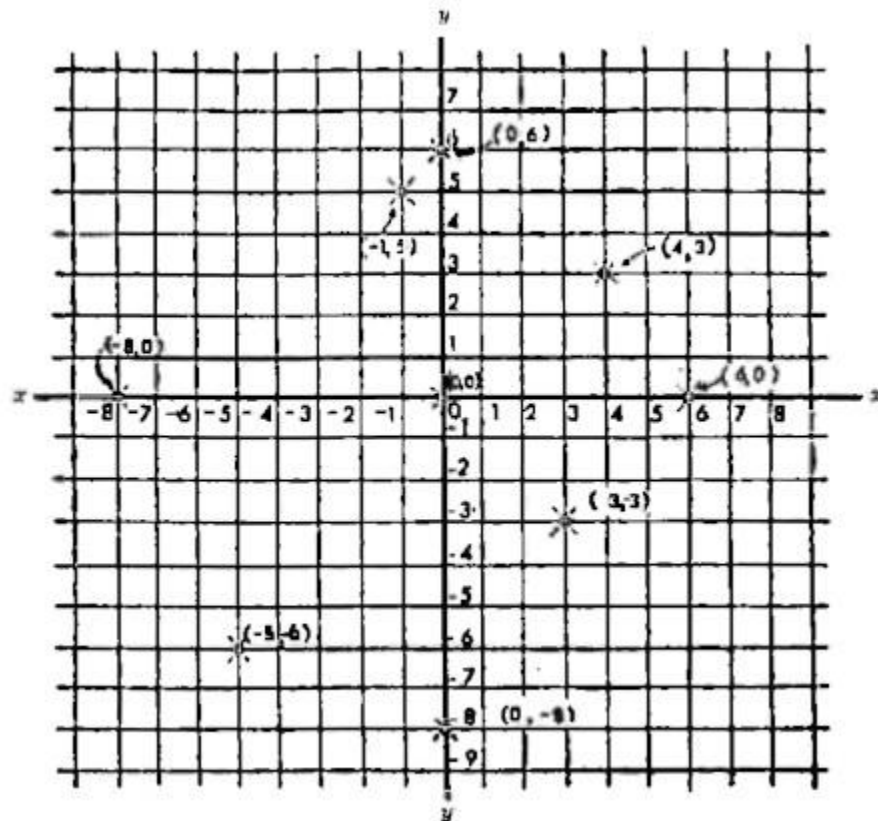
Figura 21. Los ejes de coordenadas en el plano real.
