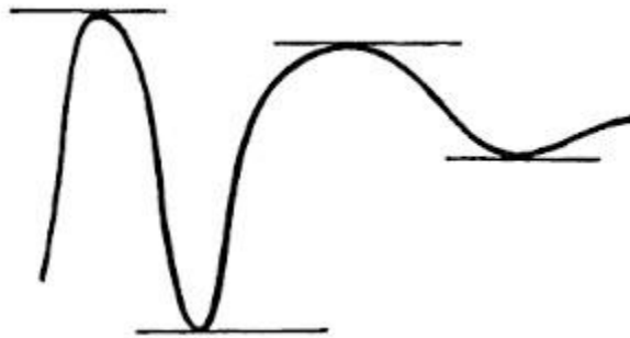
Figura 124. Las líneas horizontales son tangentes en los máximos y mínimos relativos de la curva.
