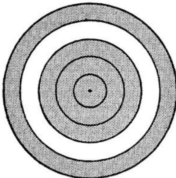
Figura 73. Las dos regiones sombreadas tienen la misma área.
