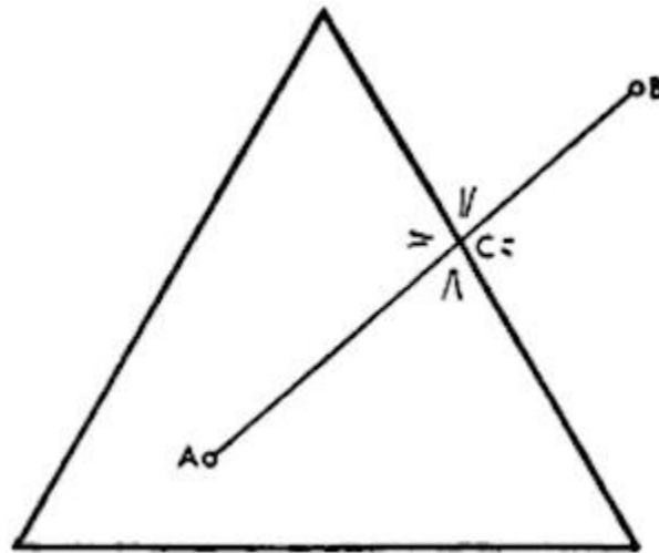
Figura 90. La línea que une el punto interior A con el punto exterior B corta al triángulo en C. No importa cómo ha sido trazada la línea: debe cortar al triángulo en algún punto.
