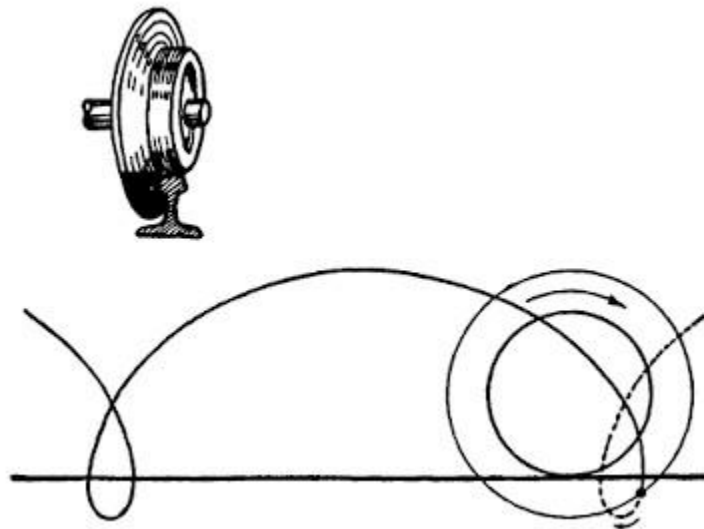
Figura 68. La cicloide alargada. Un punto perteneciente a la pestaña de una rueda de ferrocarril, en movimiento, da origen a esta curva. La parte del tren que se mueve hacia atrás cuando el tren marcha hacia delante es la porción sombreada de la rueda.
