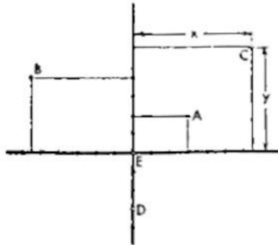
Figura 28(a). Una variedad de dos dimensiones. Cada punto requiere un par de números para ser individualizado: A = 3, 2 ; B = (-5 \frac{1}{2}, 4) ; C = (x, y) ; D = (0, -3) , E = (0, 0)
