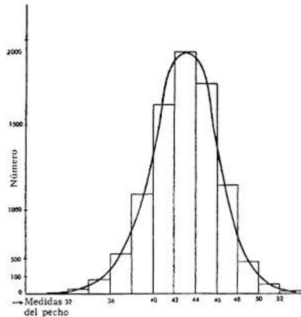
Figura 82. Esta curva de distribución indica las medidas de los perímetros torácicos de soldados escoceses. Incidentalmente sirve también para describir fenómenos tan variados como los siguientes: 1. Distribución de las edades de los jubilados de una gran empresa. 2. Jugadas en la ruleta. 3. Distribución de los impactos en el tiro al blanco.
