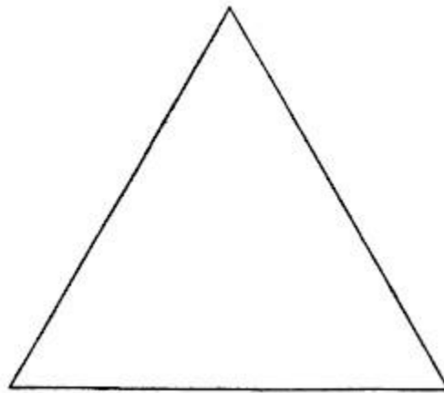
Figura 145. La primera etapa de la curva copo de nieve, C_1 .
