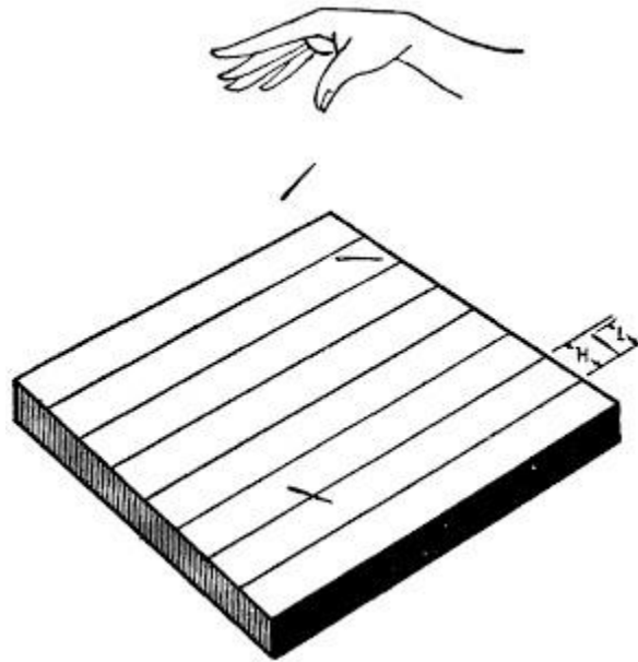
Figura 79. Problema de la aguja del conde Buffon.
