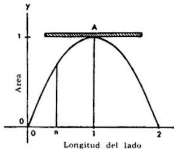
Figura 123. Esta curva es una parábola que representa las áreas de todos los rectángulos cuyo perímetro tiene una longitud igual a 4 unidades. Levántese una perpendicular en cualquier punto n del eje de las x , que llegue hasta la curva. La longitud de esta perpendicular será el área del rectángulo, uno de cuyos lados es igual a n . El área máxima corresponde al punto A de la gráfica, es decir, a la
