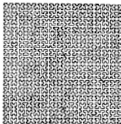
Fig. 162. Una etapa adelantada.
