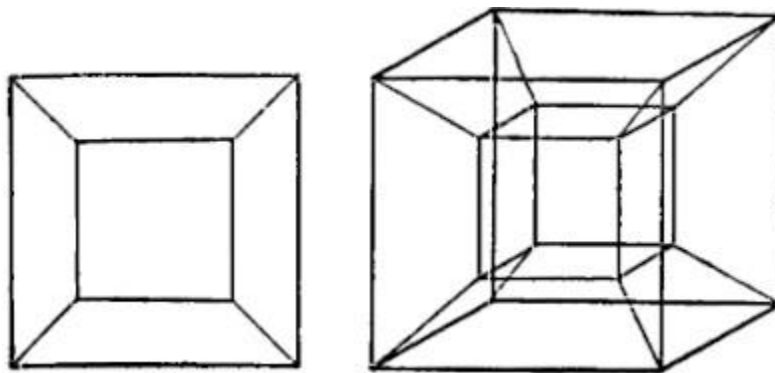
Figura 31(a). El cubo y el tesseract
