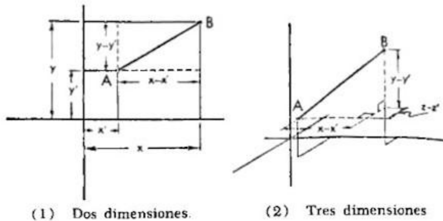
Figura 31. (1) Distancia AB = \sqrt{(x - x')^2 + (y - y')^2} ; (2) Distancia
