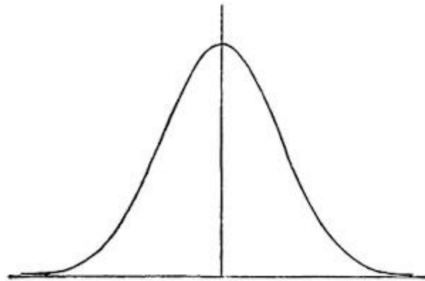
Figura 80. Curva normal de la probabilidad.
