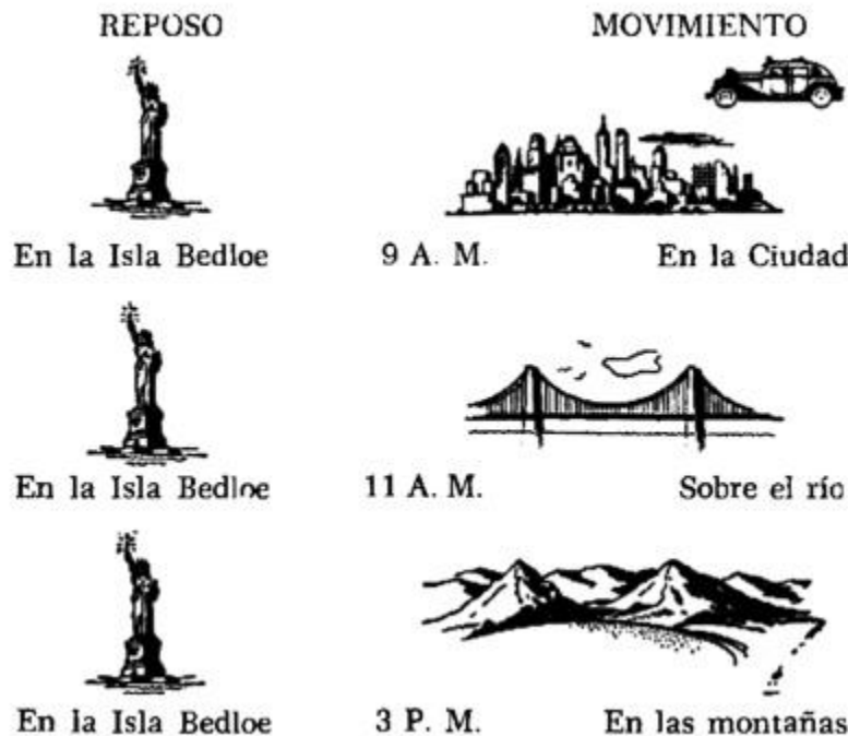
Figura 14. En los tiempos indicados, la Estatua de la Libertad está en el punto señalado, mientras que los pasajeros del taxi contemplan los distintos paisajes de la derecha.
