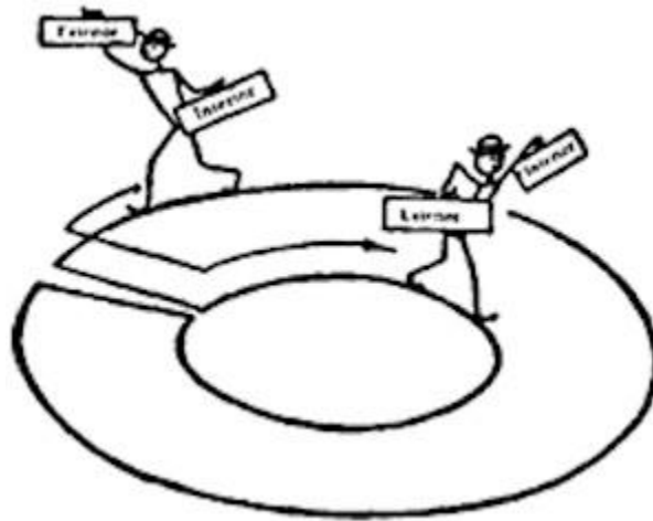
Figura 100. Interior y exterior del anillo cortado.
