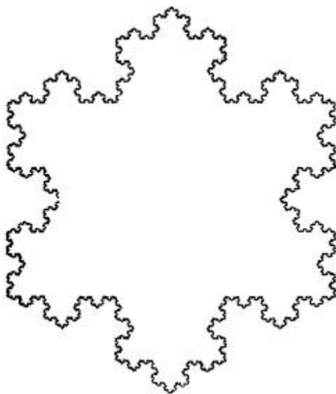
Figura 150. La sexta etapa C_6
