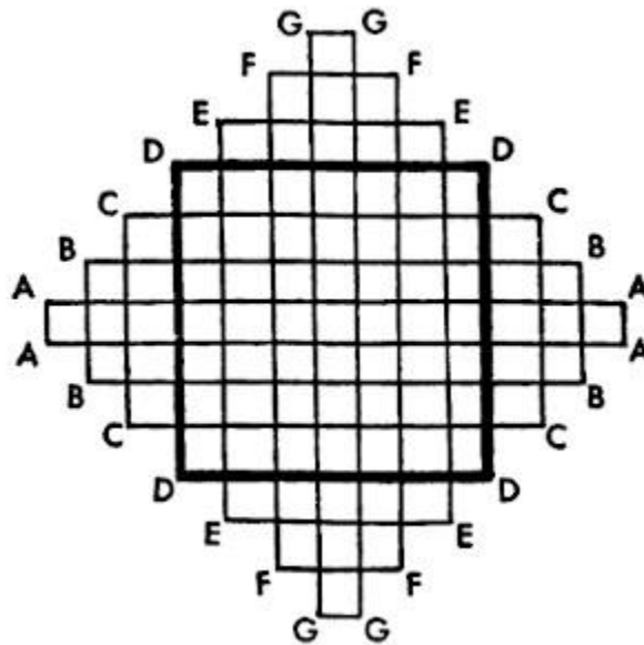
Figura 122. El perímetro de cada uno de los siete rectángulos: AAAAA, BBBBB, CCCCC, etc., es el mismo. Pero, evidentemente, el rectángulo de área máxima es el cuadrado DDDD.
