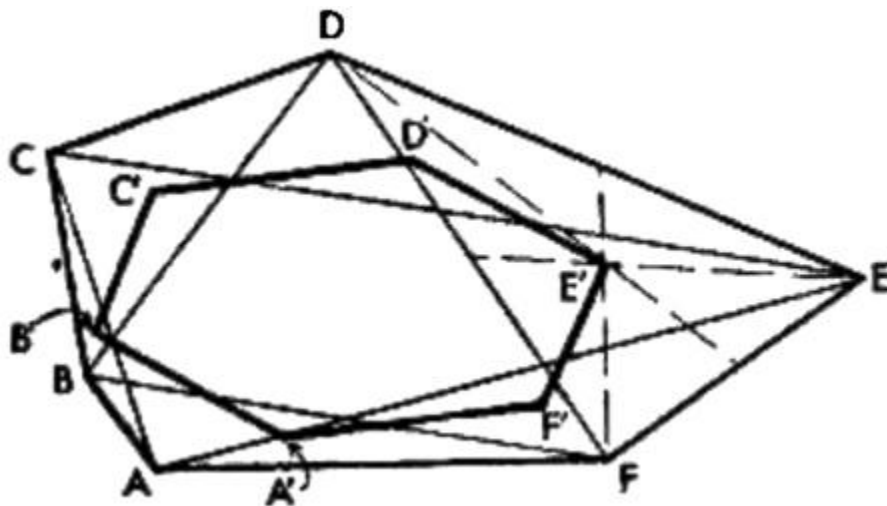
Figura 8. ABCDEF es un hexágono irregular es un parhexágono.
