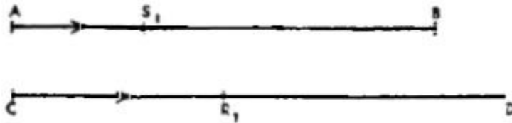
Figura 19. Interpretación dinámica de Napier de los logaritmos.
