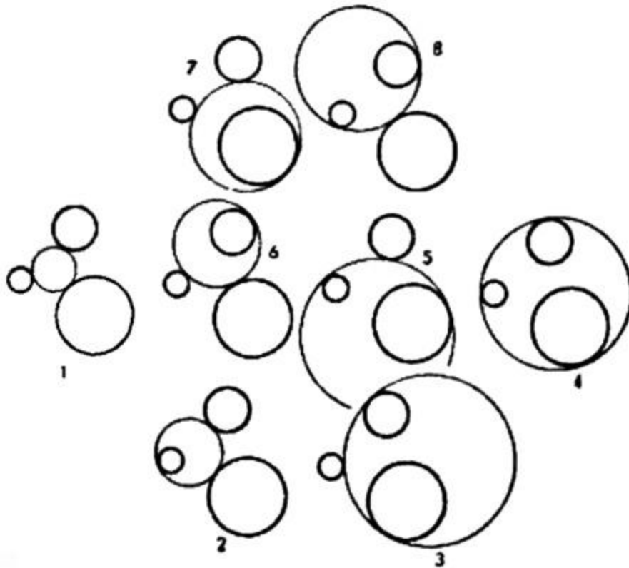
Figura 6(a). Las ocho soluciones del problema de Apolonio. Cada círculo en trazo fino es tangente a los otros tres dibujados con un trazo más grueso.
