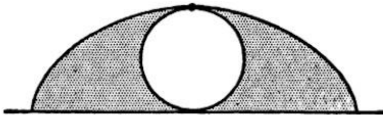
Figura 66. Cuando el círculo rodante se encuentra en la posición indicada, las superficies sombreadas que quedan a cada uno de sus lados son exactamente iguales al área del círculo.
