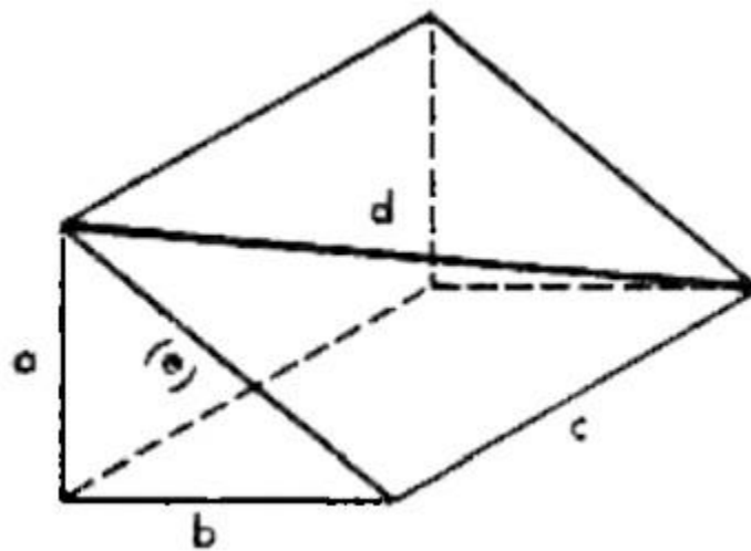
Figura 30. El teorema de Pitágoras en tres dimensiones, d^2 = a^2 + b^2 + c^2 . Pues: d^2 = c^2 + (e)^2 y (e)^2 = a^2 + b^2
