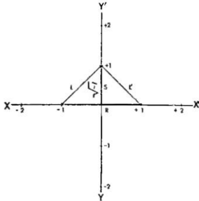
Figura 24. Interpretación geométrica de i .
