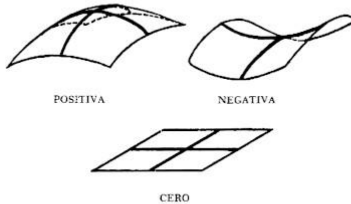
Figura 48. Curvatura.
