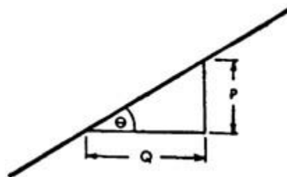
Figura 169. La pendiente de una línea recta es la razón: P/Q.
