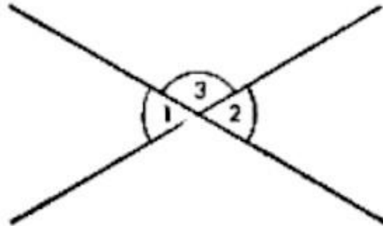
Figura 41. Ángulo 1 = ángulo 2 (porque cada uno es igual a 180^\circ menos el ángulo 3).
