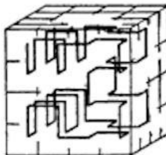
Figs. 163, 164. Las primeras dos etapas de una curva que llena en su totalidad una caja cúbica.
