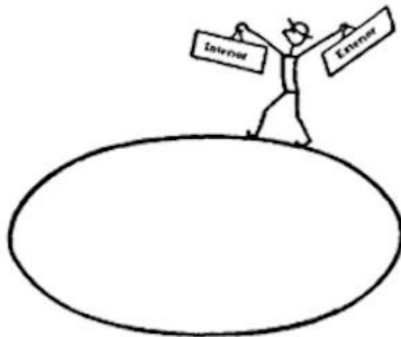
Figura 99. El hombre marcha en sentido contrario al avance de las manecillas del reloj sobre el contorno de la curva. A la izquierda queda el interior y a la derecha el exterior.
