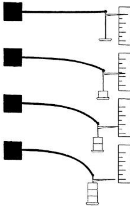
Figura 119. Cada aumento de peso flexiona la varilla un poco más.
