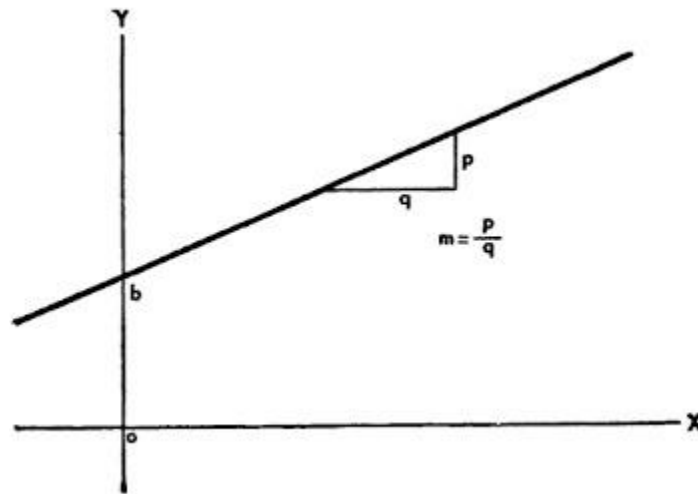
Figura 133. Representación de la ecuación: y = mx + b .
