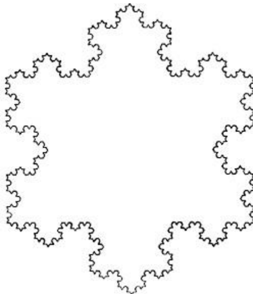
Figura 149. La quinta etapa C_5
