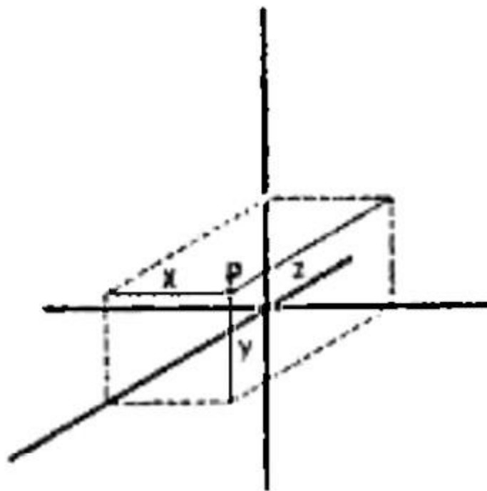
Figura 28(b). El mismo concepto puede hacerse extensivo a una
