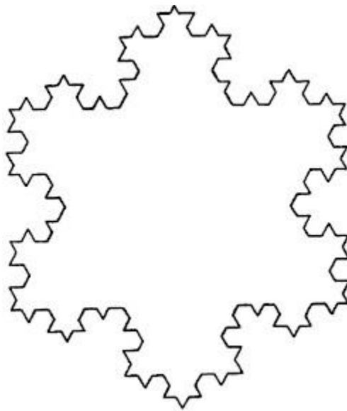
Figura 148. La cuarta etapa C_4
