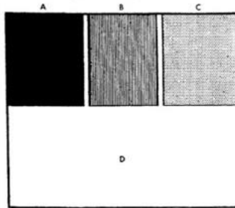
Figura 114. Los países A, B y C están separados por corredores no ocupados y D es una tierra no reclamada.
