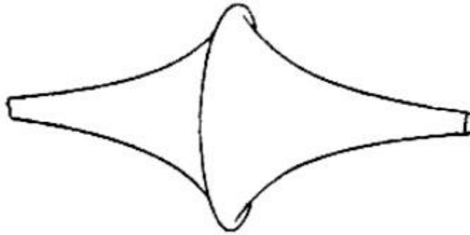
Figura 44. La pseudoesfera.
