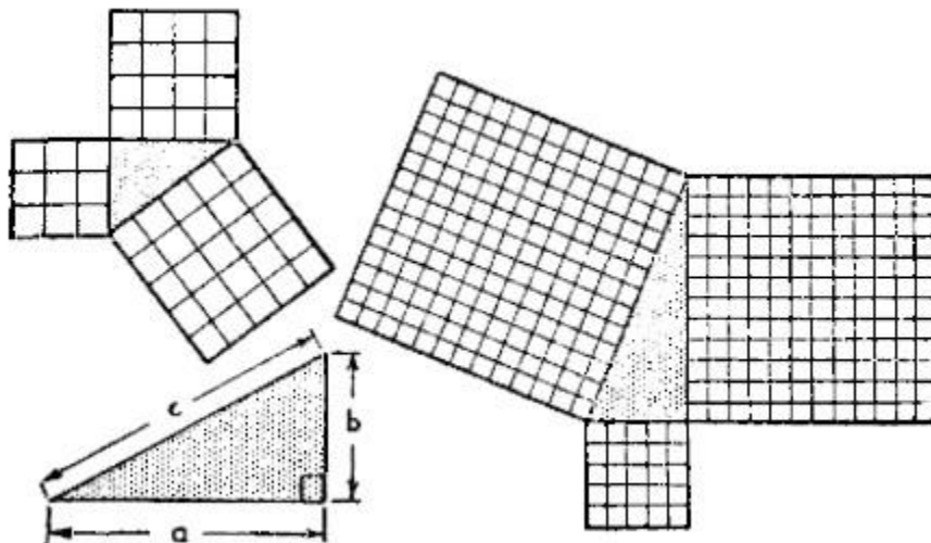
Figura 29. El teorema de Pitágoras. En todo triángulo rectángulo: c^2 = a^2 + b^2 ; o sea 5^2 = 3^2 + 4^2 ; 13^2 = 12^2 + 5^2
