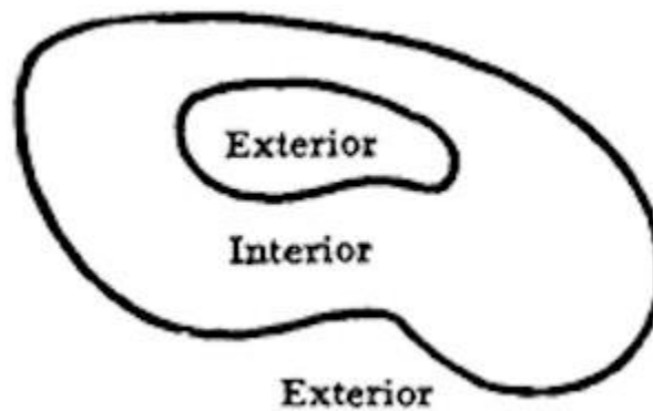
Figura 97. Ni tampoco ésta
