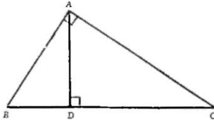
Figura 23. Longitud AD = \sqrt{(BD \times DC)} media geométrica de BD y DC .
