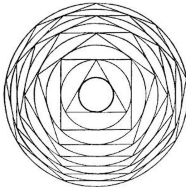
Figura 126. Los radios, al aumentar, tienden a un límite, aproximadamente 12 veces mayor que el del círculo original.
