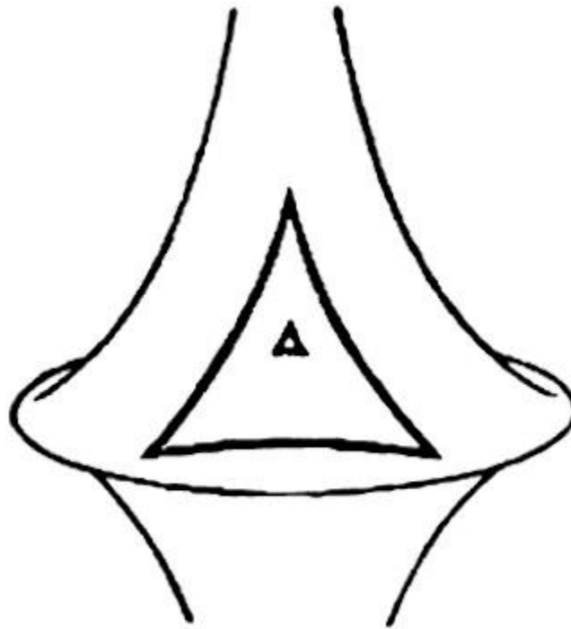
Figura 47(b). Esto es lo contrario de lo que ocurre en una esfera, figura 47(a). En una pseudoesfera, a medida que el triángulo crece, resulta menor la suma de sus ángulos.
