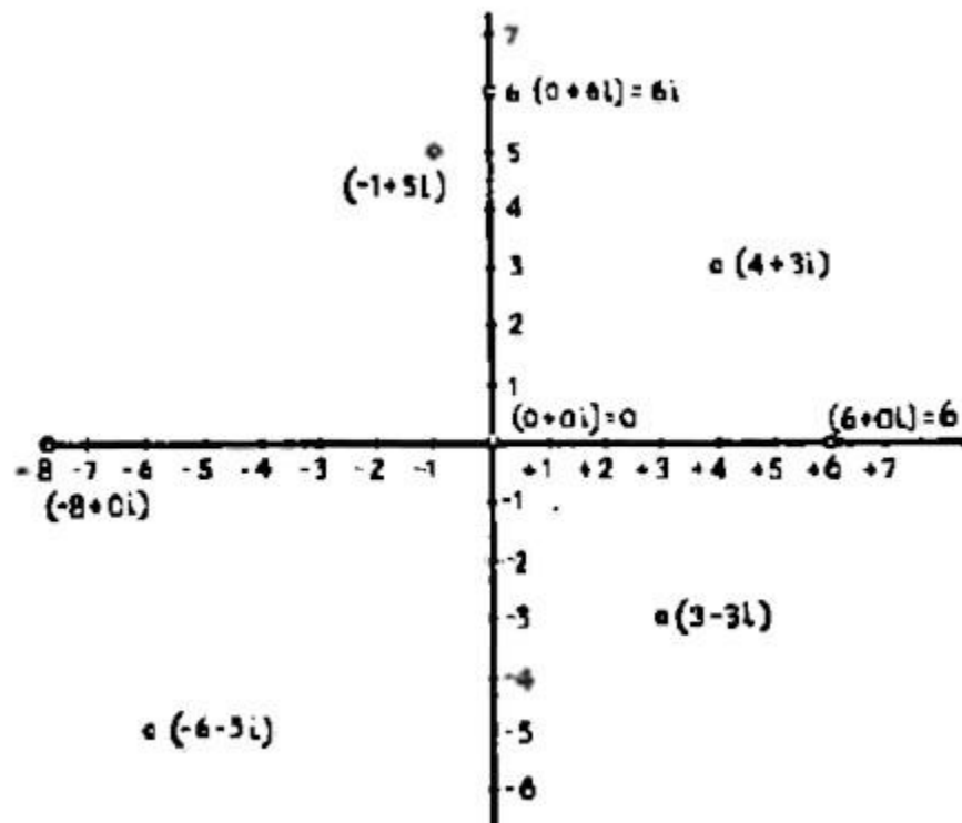
Figura 26. El plano complejo
