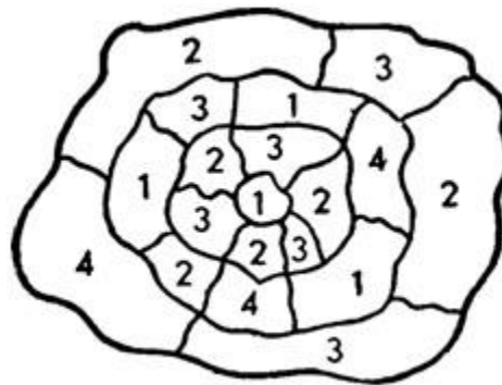
Figura 112. Una isla con diecinueve países. Solamente bastan cuatro colores para su correspondiente mapa.
