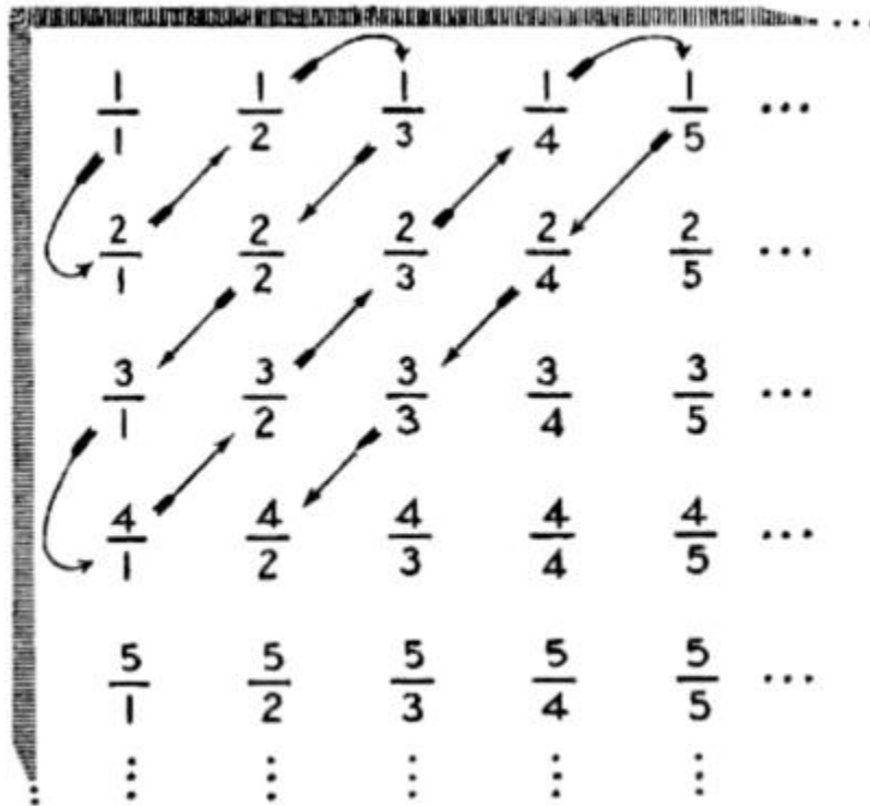
Figura 12. Método diagonal de Cantor.
