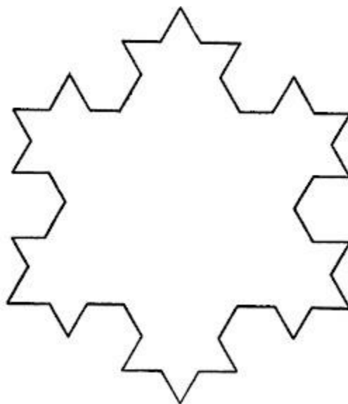
Figura 147. La tercera etapa, C_3 .
