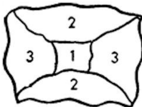
Figura 111. Una isla que es propiedad de cinco países requiere sólo de tres colores para pintar su mapa.
