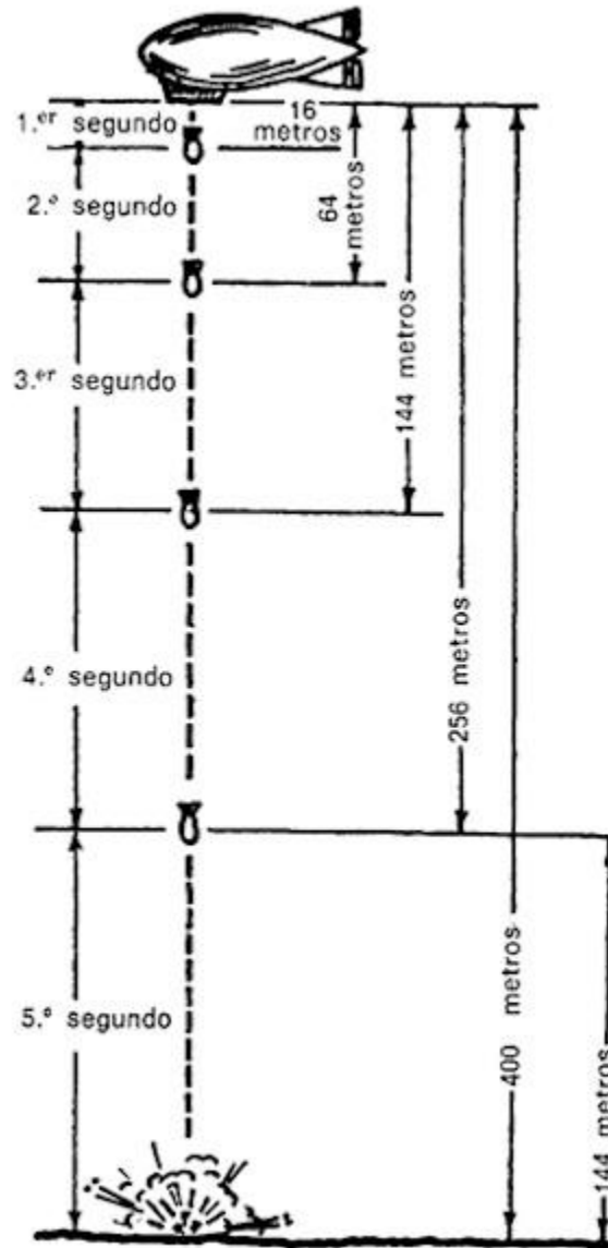
Figura 129. El dibujo muestra la distancia recorrida por un proyectil que cae, al final del 1°, 2°, 3°, 4° y 5° segundos.
