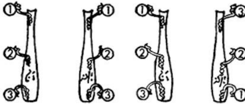
Figura 93. Únase 1 con 1, 2 con 2 y 3 con 3 mediante líneas que no se corten. Figura 94. Trátese de unir dos números correspondientes por medio de rectas que no se corten.
