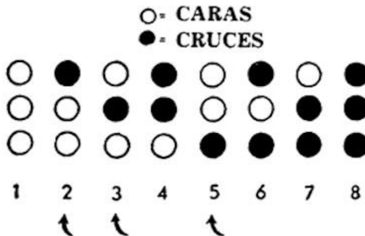
Figura 77. Los resultados posibles de tirar tres veces una moneda. Las flechas indican los casos en que se producen dos caras y una cruz.
