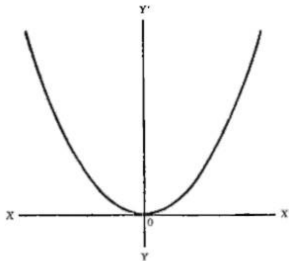
Figura 22(a). Representación gráfica de la ecuación, y = x^2 .
