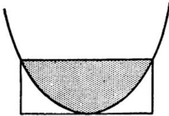
Figura 134. Cuadratura de la parábola. La superficie sombreada es igual a 2/3 del área del rectángulo.
