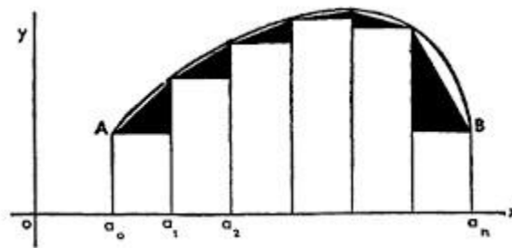
Figura 136. Aproximándose a la longitud de una curva mediante las hipotenusas de triángulos rectángulos. La base de cada triángulo es \Delta x y su altura \Delta y .
