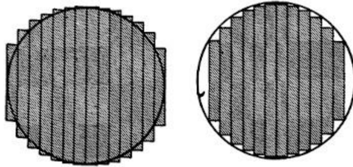
Figura 138. Aproximación del área de un círculo mediante rectángulos.
