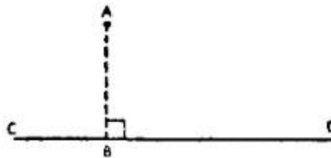
Figuras 42 y 43. Si AB = AC , entonces el ángulo 1 = ángulo 2. Desde el punto A puede trazarse una y sólo una perpendicular a CD
