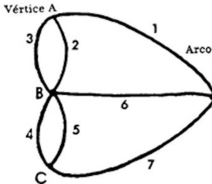
Figura 84. Una gráfica con cuatro vértices y siete arcos, correspondiente a los puentes de Königsberg.
