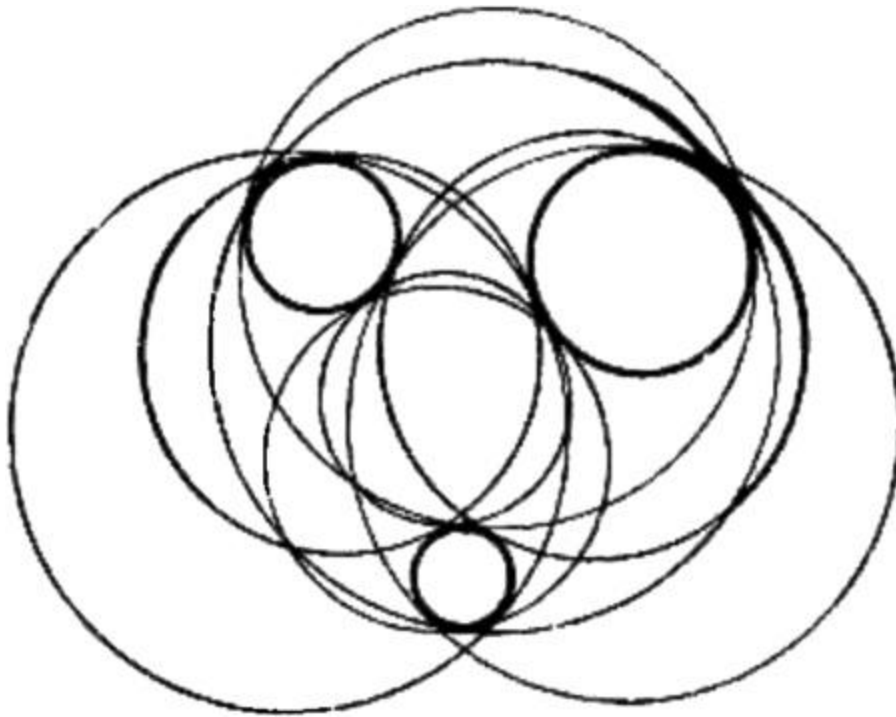
Figura 6(b). Las ocho soluciones de Apolonio reunidas en un solo diagrama.
