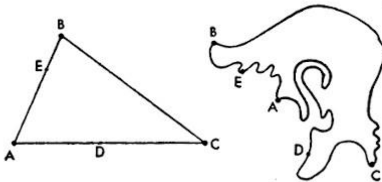
Figuras 91 y 92. Un triángulo plano. Su gemelo surrealista.
