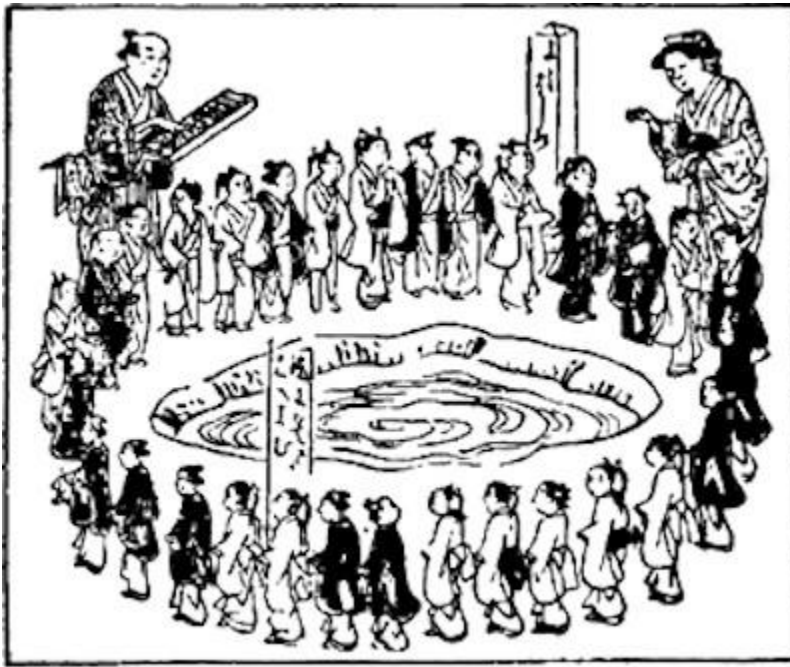
Figura 56. El problema de Josefo, de la obra Shojuisu de Miyake Kenryu. (Tomado del libro A History of Japanese Mathematics de Smith y Mikami.)
