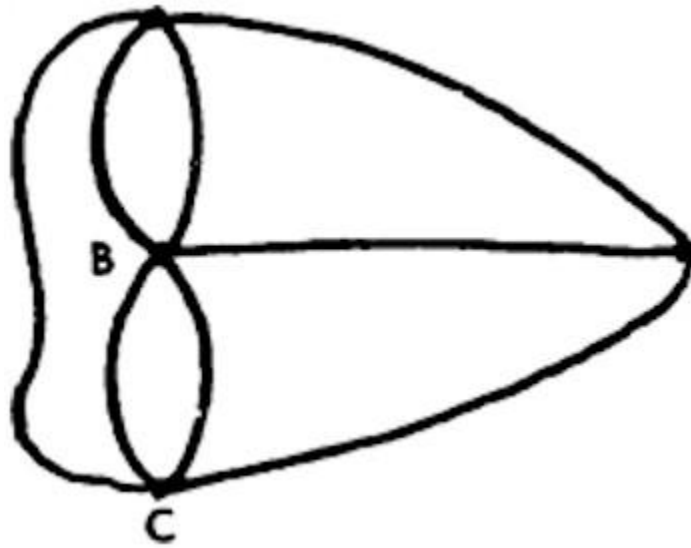
Figura 85. Una gráfica con cuatro vértices y ocho arcos.
