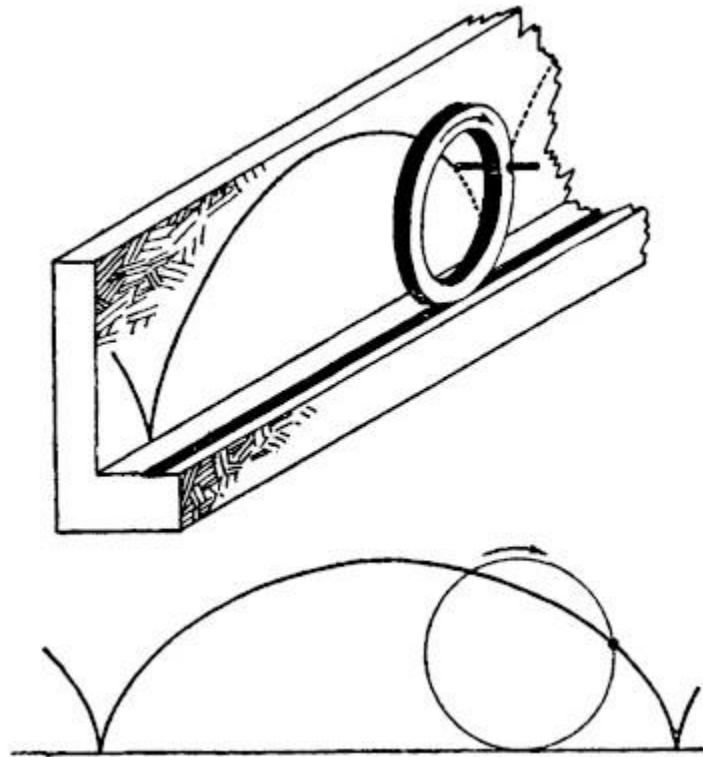
Figura 64. La cicloide.
