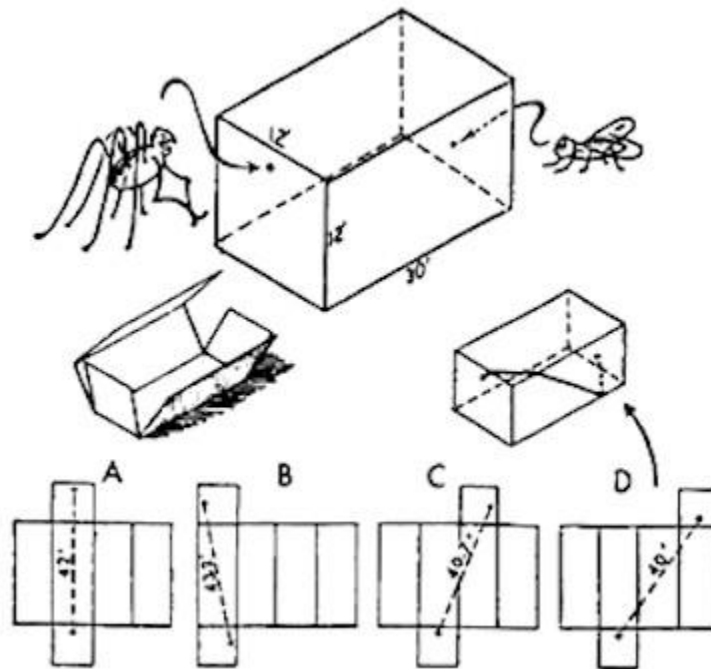
Figura 61. Habiendo la mosca rechazado su cordial invitación, la araña se pone en marcha para almorzar siguiendo la ruta más corta posible. ¿Qué trayectoria representa la geodésica para la famélica araña?
