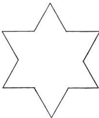
Figura 146. La segunda etapa de la curva copo de nieve, C_2 .
