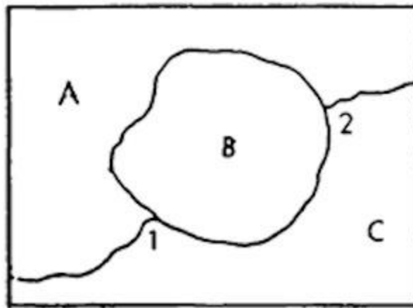
Figura 113. Los puntos 1 y 2 son comunes a los tres países A, B, C.
