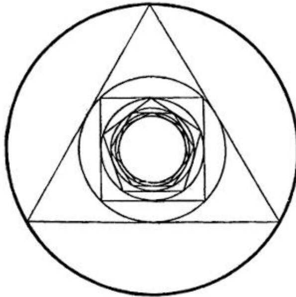
Figura 125. Los radios, al disminuir, tienden a un límite, que es aproximadamente 1/12 del valor correspondiente al radio del primer círculo.
