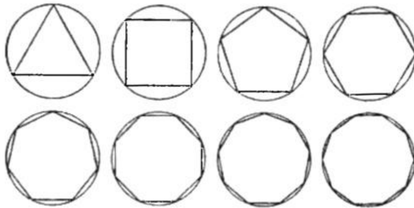
Figura 4. El círculo como límite de polígonos inscritos.
