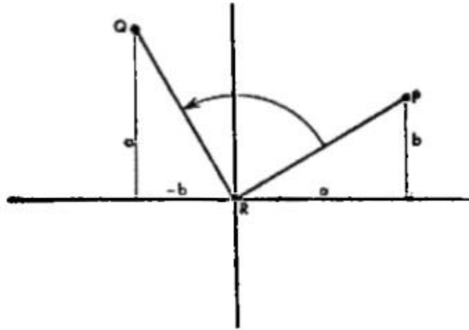
Figura 25. La multiplicación por i es una rotación de 90^\circ . Sea P = (a + ib) , entonces P \times i = (a + ib) \times i = (a \times i) + (b \times i \times i) = ia + b \times -1 = -b + ia = 0
