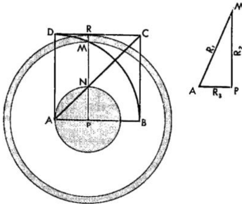
Fig. 11. Sustráigase el triángulo APM de la figura. Es fácil ver que sus tres lados son iguales, respectivamente, a los radios de los tres círculos. Luego: R_1^2 - R_2^2 = R_3^2 , o bien: \pi R_1^2 - \pi R_2^2 = \pi R_3^2 ; o bien: las dos superficies sombreadas son iguales.
