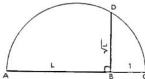
Fig. 27. Sea AB la longitud dada. Extiéndasela hasta C de manera que BC = 1 . Trácese un
