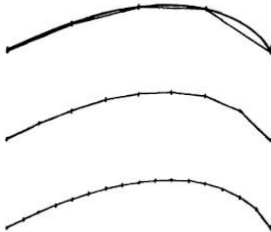
Figura 135. Aproximándose a la longitud de una curva mediante segmentos rectilíneos.
