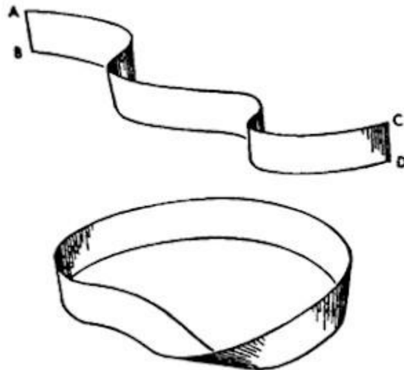
Figuras. 103 y 104. La cinta de Möbius, una superficie unilátera y bilátera.
