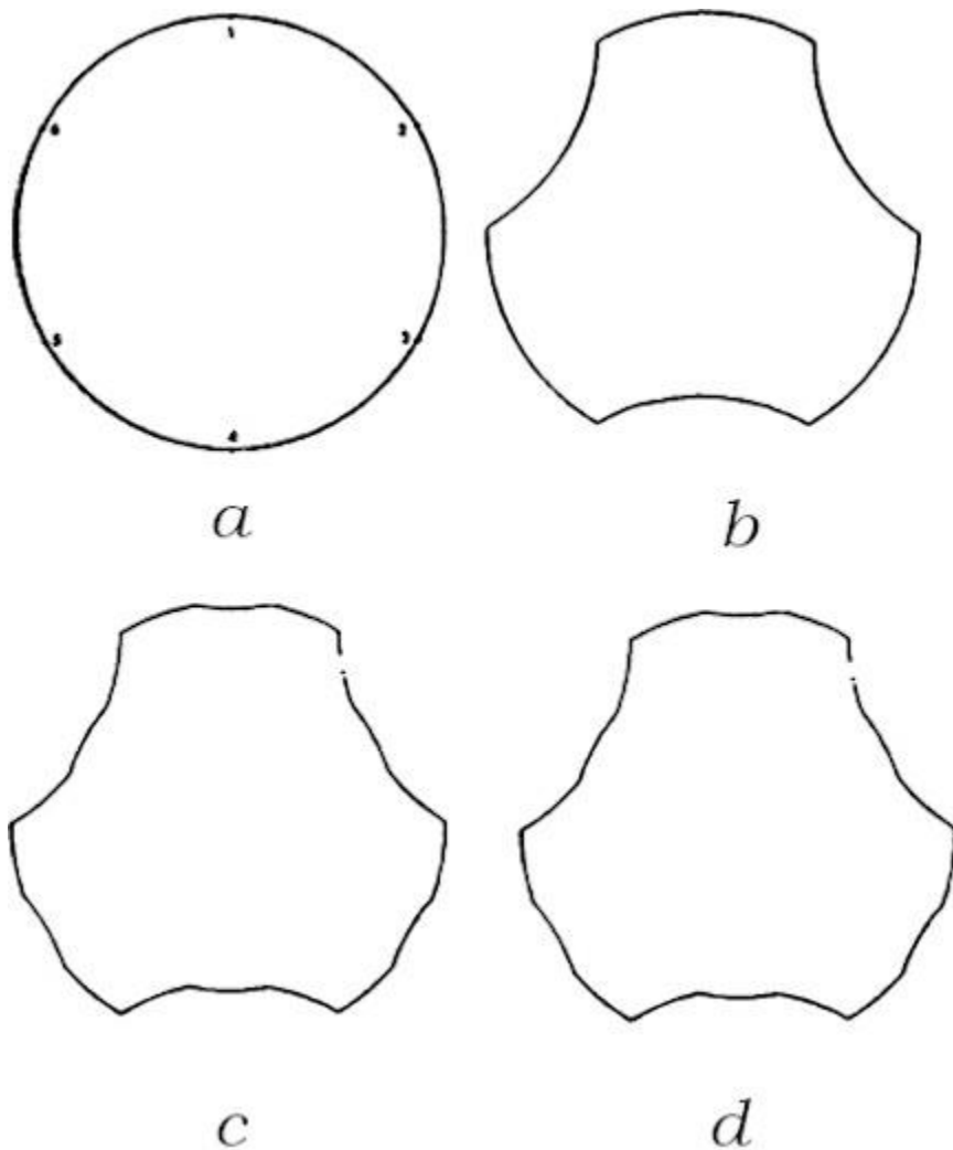
Figuras 155-158. (a) La curva que entra y sale, etapa C_1 . (b) Etapa
