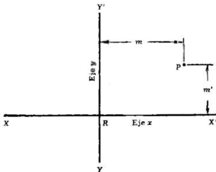
Figura 20. El punto P tiene las coordenadas (m, m')
