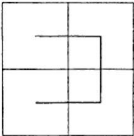
Fig. 159. La curva que llena el espacio. Etapa 1.
