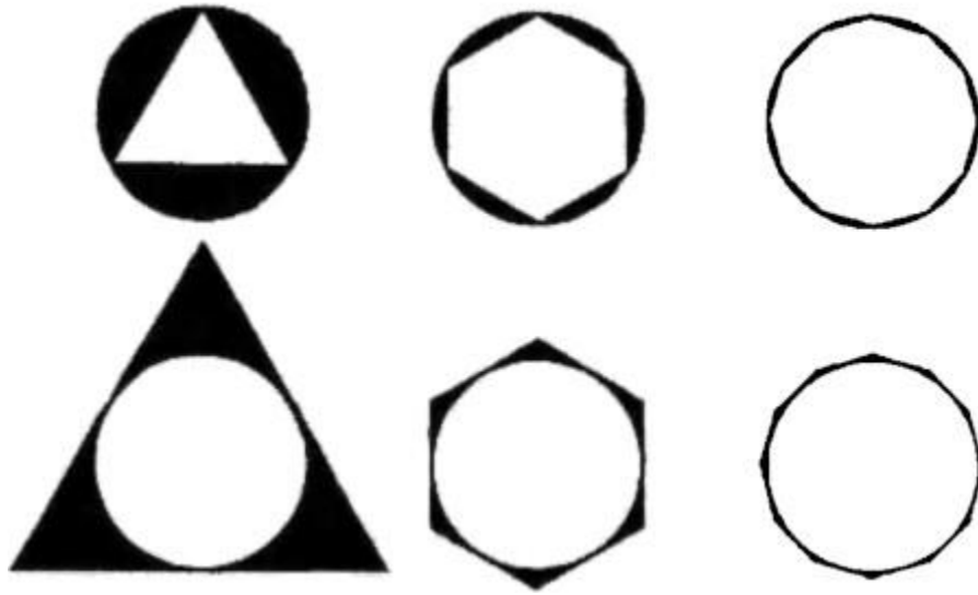
Figura 16. El círculo como límite de polígonos inscritos y circunscritos.
