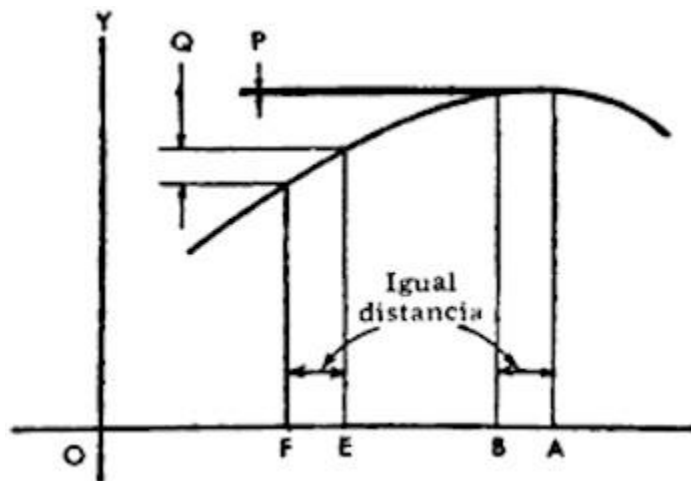
Figura 120. La razón de cambio de una cantidad variable es más pequeña en el punto máximo que en cualquier otra parte.
