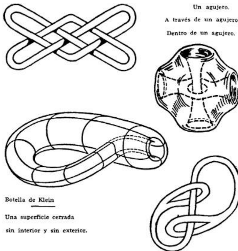
Figura 102. Variedades topológicas rarísimas. Complicaciones derivadas de las rosquillas.
