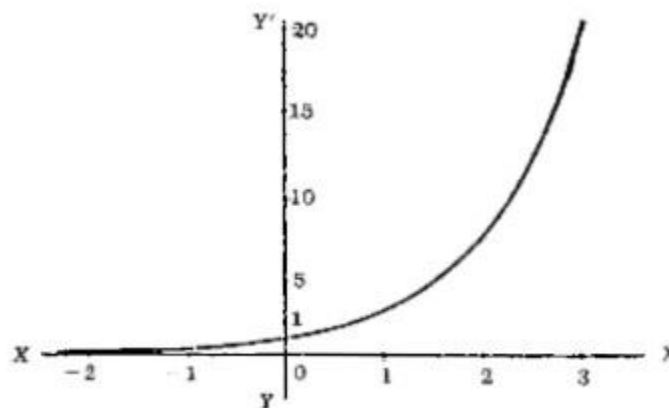
Figura 22(c). Representación gráfica de la ecuación: y = e^x . Esta curva muestra la propiedad común a todos los fenómenos de crecimiento: la razón de crecimiento es proporcional al estado de crecimiento.
