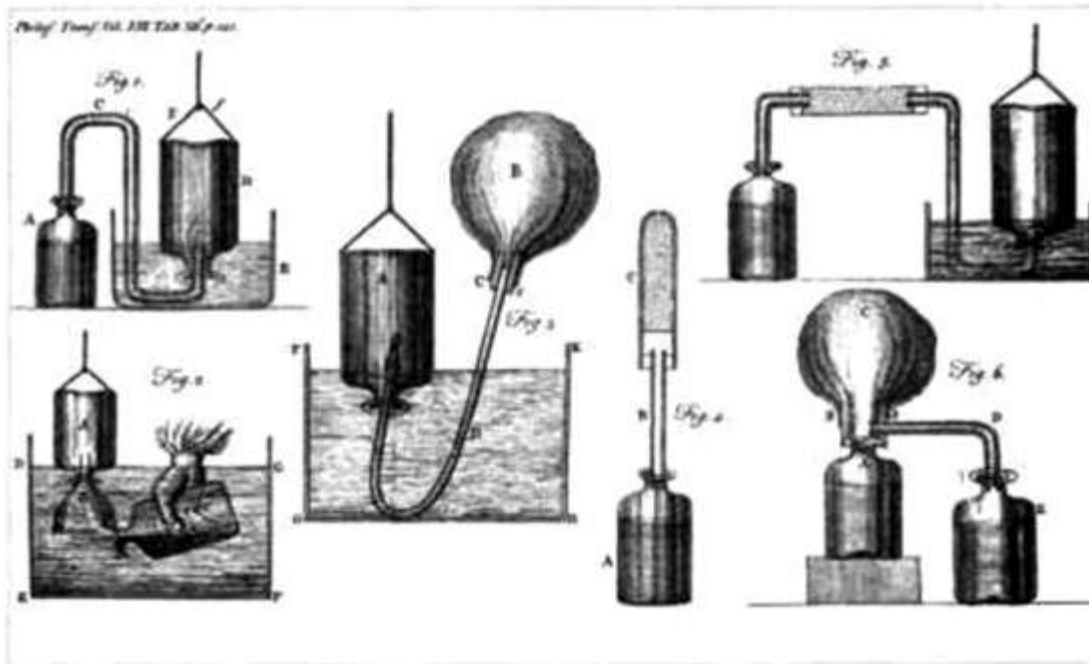
Lámina que acompañaba el artículo «Three Papers, Containing Experiments on Factitious Air» (1766) para ilustrar los diferentes experimentos que había realizado sobre el aire facticio.
