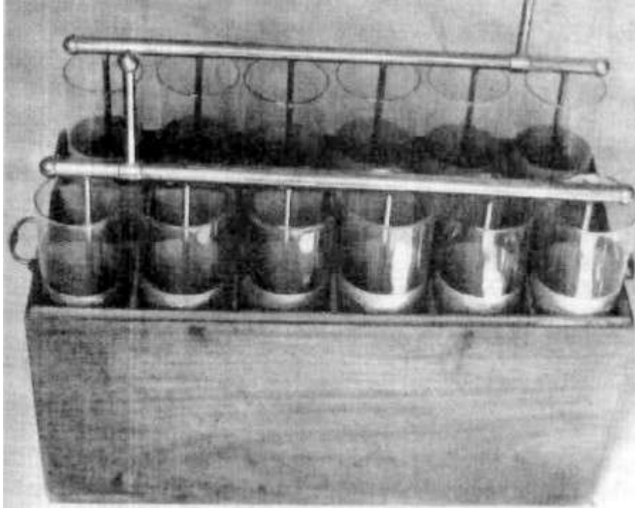
Batería de botellas de Leiden que usó Cavendish en sus experimentos para aumentar la cantidad de electricidad disponible.
