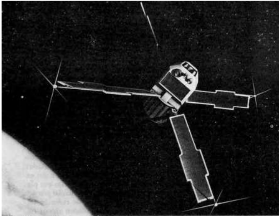
Figura 10-1. El satélite de rayos X Uhuru dibujado en el espacio. Los cuatro “paneles solares” proporcionan energía solar a los aparatos. Los receptores de rayos X del cuerpo principal del satélite exploran el cielo por bandas mientras éste gira alrededor de su eje cada diez minutos. Los resultados de las mediciones se envían por radio a la Tierra.
