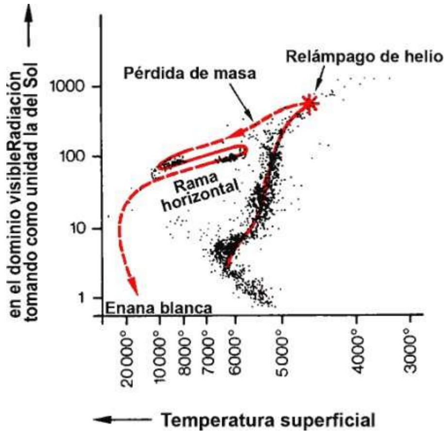
Figura 7-2. Trayectoria evolutiva esquemática de una estrella de tipo solar en el diagrama HR. La estrella después de pasar por la secuencia principal se convierte en una gigante roja, como indicaba la figura 5-4. Su helio entra entonces en ignición (relámpago de helio). La explosión proyecta al espacio tanta cantidad de su materia que desaparece una parte esencial de la envoltura de la gigante roja y la estrella llega así a la rama horizontal del diagrama. Luego se convierte probablemente en una enana blanca. Se han dibujado como comparación en el diagrama las estrellas del cúmulo estelar M3 de la figura 2-9.
