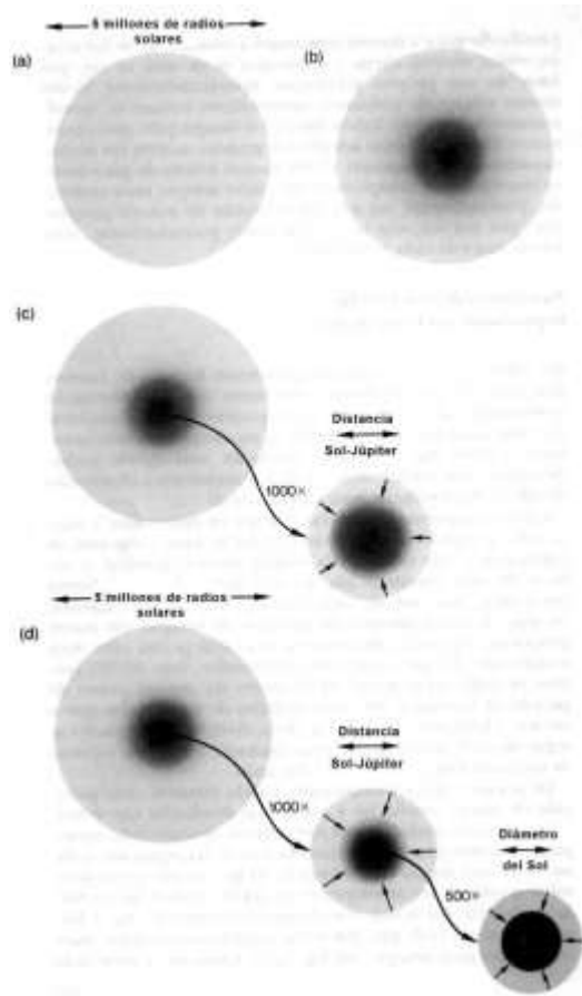
Figura 12-2. Modelo de Larson sobre el nacimiento del Sol. (a) Una nube de gas interestelar empieza a contraerse. Al principio, la densidad de su interior es idéntica en todas partes, (b) Al cabo de 390.000 años, la densidad en el centro de la nube se ha centuplicado, (c) Pasados 423.000 años desde el inicio del proceso aparece en el interior de la condensación neutral un núcleo caliente, que al principio no se contrae más. Está representado en el dibujo a escala ampliada. Su densidad es diez millones de veces superior a la densidad inicial. La masa principal continúa situada en la nube que rodea este núcleo y que prosigue su contracción. (d) Poco después, cuando en el núcleo las moléculas de hidrógeno se disocian dando átomos individuales, el núcleo se contrae de nuevo y forma un nuevo
