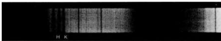
Figura A-1. Espectro de la estrella 41 Cygni, registrado por Waltraut
