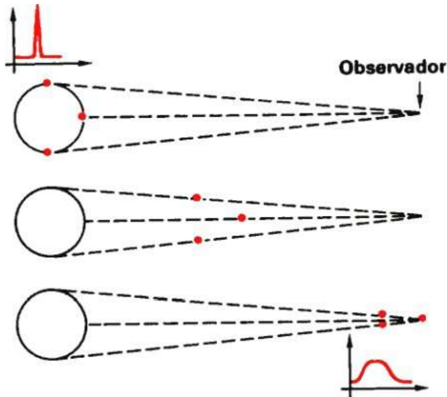
Figura 8-3. El impulso de luz (arriba a la izquierda) emitido por una superficie esférica se alarga y difumina en el tiempo para un observador lejano (derecha, arriba y abajo), porque las señales luminosas procedentes de puntos distintos de la esfera tardan tiempos distintos en llegar a él.
