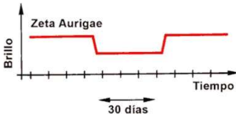
Figura 1-2. Curva de luminosidad de la estrella zeta Aurigae. La luminosidad disminuye un 65% en el intervalo de un día. Luego, la estrella permanece debilitada 37 días para volver de nuevo a su luminosidad en el curso de un día. Pasados 972 días se repite el mismo proceso.
