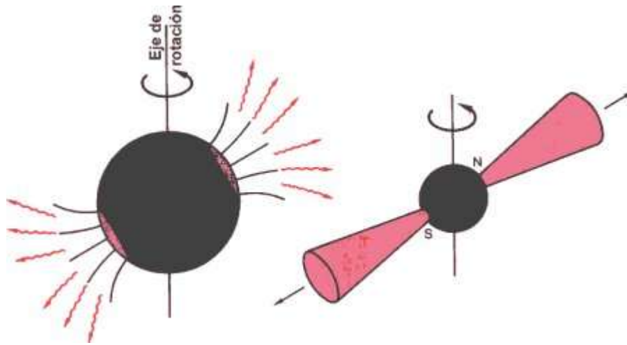
Figura 8-10. Modelo posible del origen de las señales del pulsar. Por los dos polos magnéticos N y S de una estrella de neutrones en rotación escapan electrones al espacio con una velocidad próxima a la de la luz siguiendo las líneas del campo magnético. La energía que emiten cerca de la estrella forma un haz en su dirección de fuga. Los cuantos de radiación están representados en el dibujo de la izquierda por flechas onduladas. La radiación que escapa de la estrella de neutrones sale de los polos magnéticos hacia el espacio en forma de dos conos radiantes (derecha). La rotación de la estrella de neutrones arrastra consigo estos dos conos, que iluminan el espacio como dos reflectores. Un observador sólo capta radiación cuando uno de los conos le ilumina. La rotación de la estrella de neutrones ilumina al observador siguiendo el ritmo con que ella gira.
