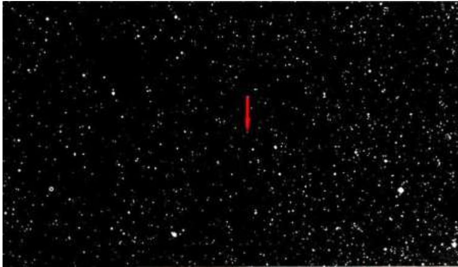
Figura 10-7. Región del cielo donde Uhuru descubrió la fuente de Hércules. La débil estrella variable de Hoffmeister está señalada con una flecha.
