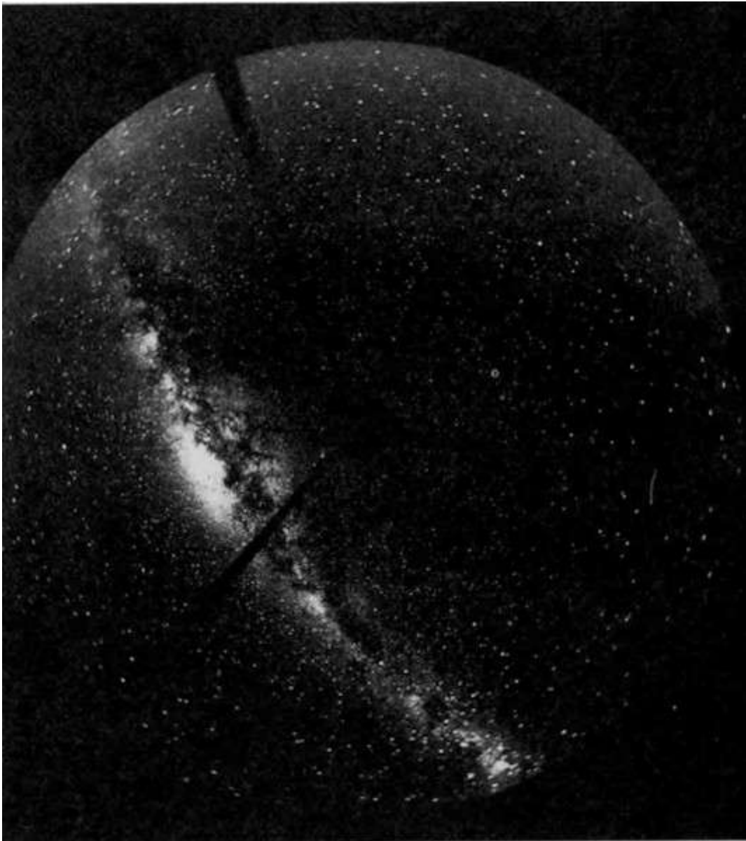
Figura 0-3. La Vía Láctea fotografiada con una cámara gran angular. Las líneas negras que cruzan la imagen se deben a la misma cámara. (Fotografía: W. Schlosser, Astron. Institut der Ruhr-Universität, Bochum.)
