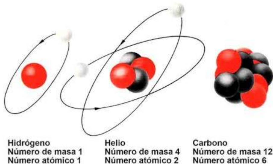
Figura 3-1. Representación esquemática de los átomos de hidrógeno, helio y carbono. Los protones están esquematizados en blanco y los neutrones en gris oscuro. Las órbitas de los electrones que giran alrededor del núcleo (dibujados en gris claro) no están a escala. No se han dibujado los seis electrones que orbitan el núcleo del carbono.
