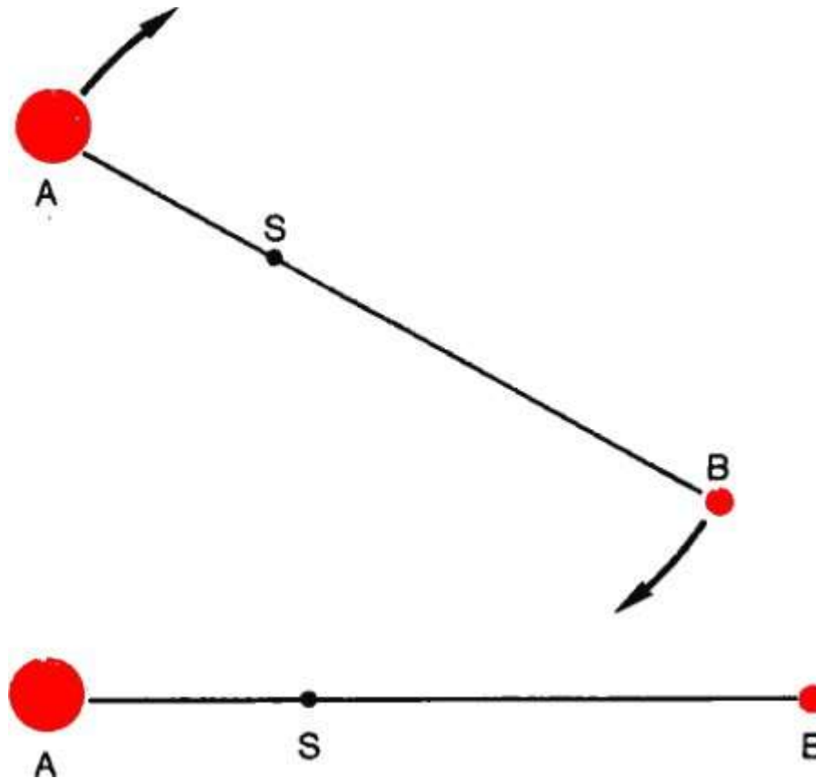
Figura C-1. Movimiento en un sistema estelar doble (simple). Arriba: Punto de mira perpendicular al plano orbital. Las dos estrellas A y B se mueven en órbitas circulares de radios distintos alrededor del centro de gravedad común S. Debajo: El mismo movimiento observado de lado. Cuando la línea que une ambas estrellas es exactamente perpendicular a la dirección del observador —como ahora en el dibujo—, una de las estrellas al moverse se acercará a nosotros, mientras la otra se alejará. Las correspondientes velocidades pueden calcularse luego mediante el efecto Doppler descrito en el Apéndice A.
