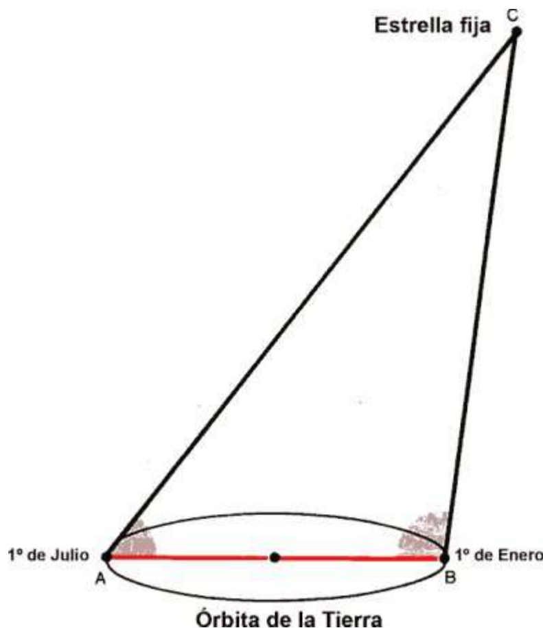
Figura B-1. Esquema de la determinación de la distancia a una
