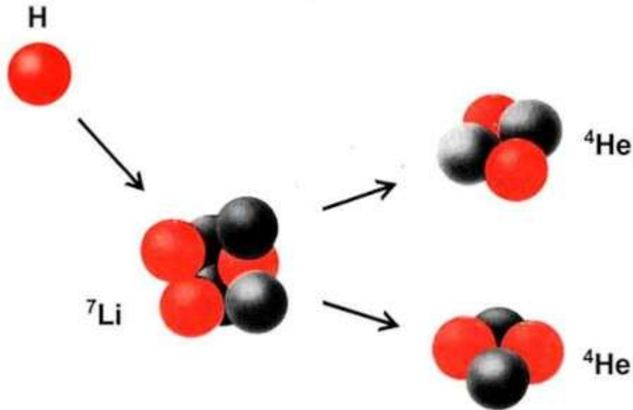
Figura 5-3. A una temperatura de tres millones de grados los átomos de litio del interior de una estrella se transforman en helio ayudados por núcleos de hidrógeno.
