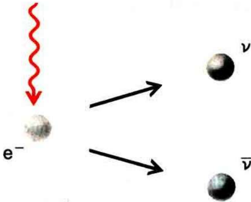
Figura 7-1. Cuando se tienen temperaturas de centenares de millones de grados, el encuentro de un electrón (esfera gris) y de un cuanto de luz (flecha ondulada) puede crear un neutrino y un antineutrino.
