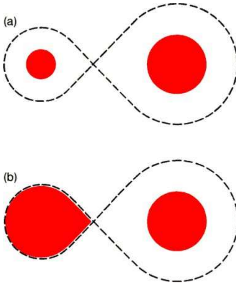
Figura 9-2. Sistema estelar doble separado (a). Ambas estrellas están situadas claramente dentro de su volumen máximo permitido, que delimitan las curvas de trazos. — Sistema doble semi separado (b). La estrella de la izquierda llena exactamente su volumen de Roche.
