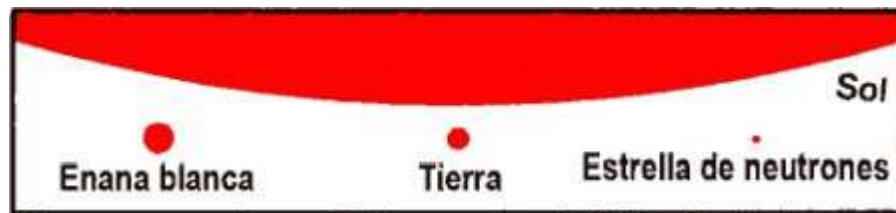
Figura 8-9. El Sol, una enana blanca, la Tierra y una estrella de neutrones comparados a escala. El Sol muestra sólo su borde en la parte superior del dibujo.
