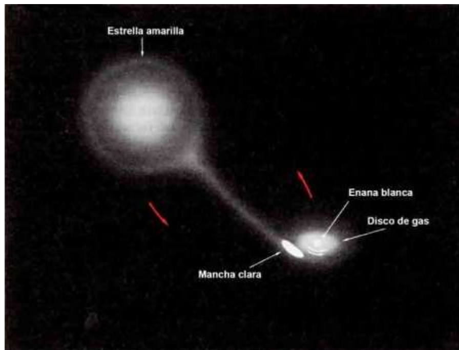
Figura, 9-8. Los dos componentes del sistema estelar doble de una nova giran uno alrededor del otro según indican las flechas exteriores. Una estrella de la secuencia principal llena su volumen máximo permitido. Gas procedente de su superficie fluye hacia la enana blanca acompañante. Pero la materia gira primero dentro de un disco antes de precipitarse sobre la enana blanca. Las flechas interiores indican el movimiento en este disco. En el punto donde la corriente de gas procedente de la estrella de la secuencia principal choca contra el disco rotatorio, se observa una mancha caliente y brillante.
