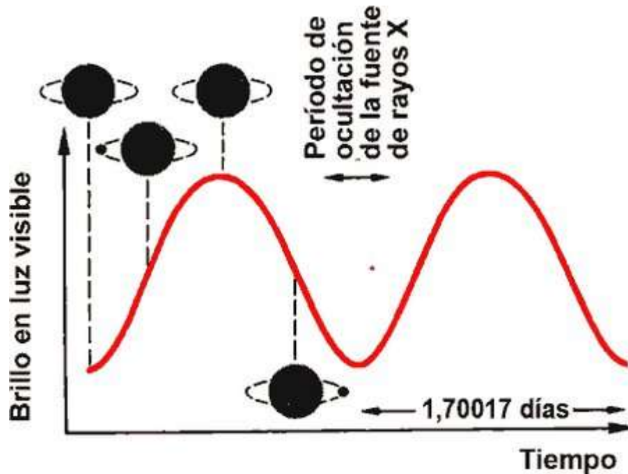
Figura 10-8. La luminosidad de la estrella variable de Hoffmeister, H2 Herculis, aumenta y disminuye regularmente (curva). En la mitad izquierda del dibujo, cuatro esquemas representan arriba y abajo de la curva las respectivas posiciones de la estrella (disco) y de la fuente de rayos X (punto), en relación al observador. Cuando la fuente de rayos X está situada delante de la estrella —desde nuestro punto de vista— vemos la cara calentada por la fuente y la estrella nos parece más brillante. Cuando la fuente está situada detrás de la estrella, sólo vemos la cara “normal” no calentada; la estrella nos parece débil.
