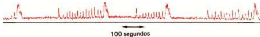
Figura 10-14. Las señales de la Fuente MXB 1730-335 proceden de un cúmulo estelar globular cuya existencia cobró interés por la presencia de la fuente de rayos X. Los impulsos llegan en forma de chubascos formados por un número de explosiones individuales que va de diez a veinte. Los impulsos no tienen siempre igual intensidad. La fuente necesita a menudo después de explosiones muy potentes una pausa de recuperación para poder emitir nuevos impulsos.
