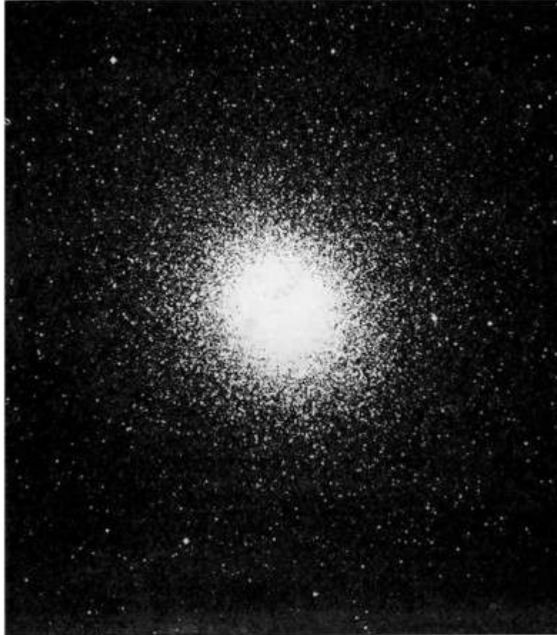
Figura 2-6. Cúmulo globular 47 Tucanae, fotografiado con el telescopio reflector Schmidt de 1 m del Observatorio Austral Europeo (ESO) en Chile. Las estrellas están tan apretadas que la fotografía no llega a resolver en estrellas individuales la zona central. Parece como si las estrellas del centro estén casi tocándose, pero en realidad su separación continúa siendo grande.
