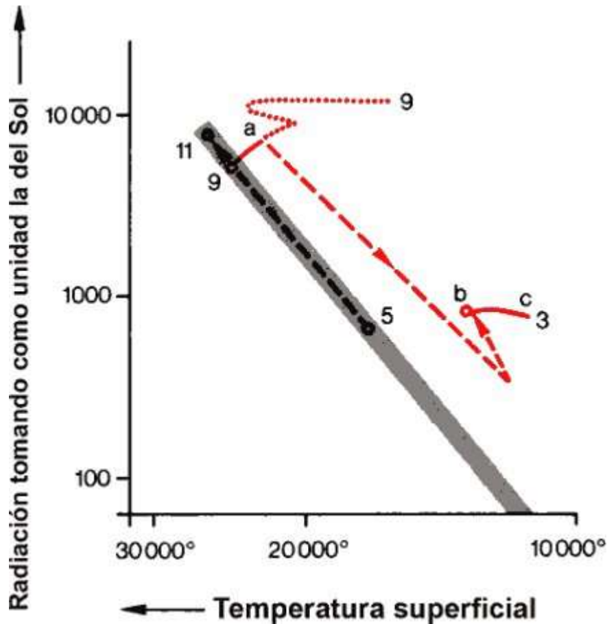
Figura 9-4. Evolución de un sistema doble compacto formado por dos componentes de 5 y 9 masas solares. El agotamiento de la reserva de hidrógeno se hace notar primero en la estrella de mayor masa.
