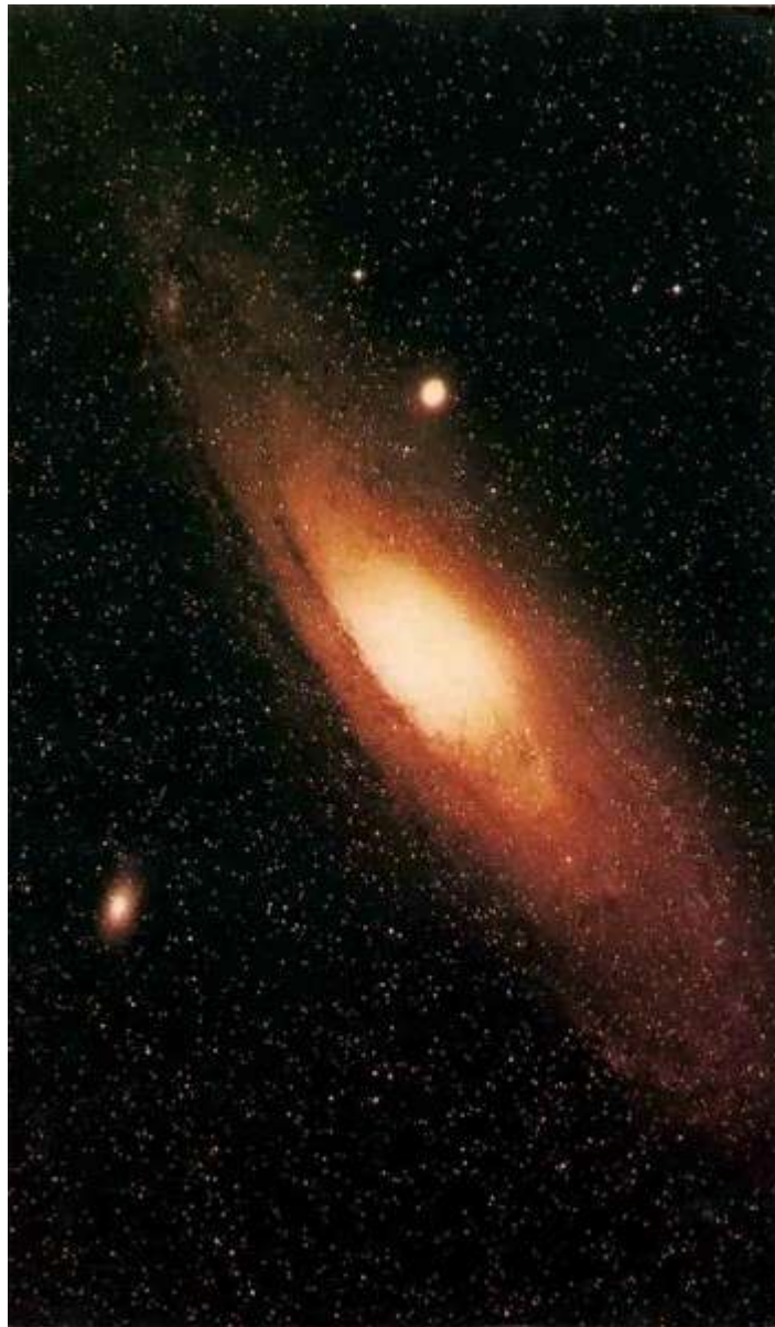
Figura 0-1. La galaxia de Andrómeda está situada a unos dos millones de años luz de nuestra galaxia Vía Láctea, a la que pertenecen todas las estrellas solas que pueden reconocerse en la fotografía. La nebulosa de Andrómeda aparece como una mancha nebulosa y elíptica. Sólo los mayores telescopios pueden resolver esta "nebulosa" en innumerables estrellas. Muchas galaxias presentan la
