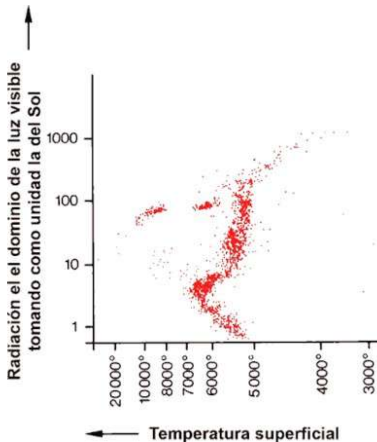
Figura 2-9. Diagrama HR del cúmulo estelar M3. Es un cúmulo globular como el de la fotografía de la figura 2-6. Sólo quedan en la secuencia principal estrellas cuya radiación es cinco veces la del Sol. La mayoría de estrellas más brillantes no pertenecen a la secuencia principal. En otras secciones de esta obra veremos la importancia que tienen, entre otras, las estrellas cuya radiación visible es cien veces superior a la del Sol y que ocupan una banda horizontal que se extiende de los 5.800 grados a los 13.000 grados. Forman la llamada rama horizontal.
