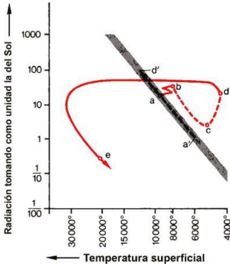
Figura 9-5. Formación de una enana blanca. La estrella de mayor masa, formada por dos masas solares, parte de a en la secuencia principal; la otra, que tiene la masa del Sol, parte de a'. La estrella de mayor masa evoluciona primero y alcanza en b su volumen de Roche. Entrega entonces masa a su acompañante y se desplaza a lo largo de la trayectoria evolutiva de trazos. En d ha finalizado ya el intercambio de masa. La estrella, que conserva solamente 0,26 masas solares, se convierte en el trayecto hacia e en una enana blanca. La estrella acompañante se desplaza por la secuencia principal con masa creciente hacia d'. Comparar este dibujo con el de la figura 9-6
