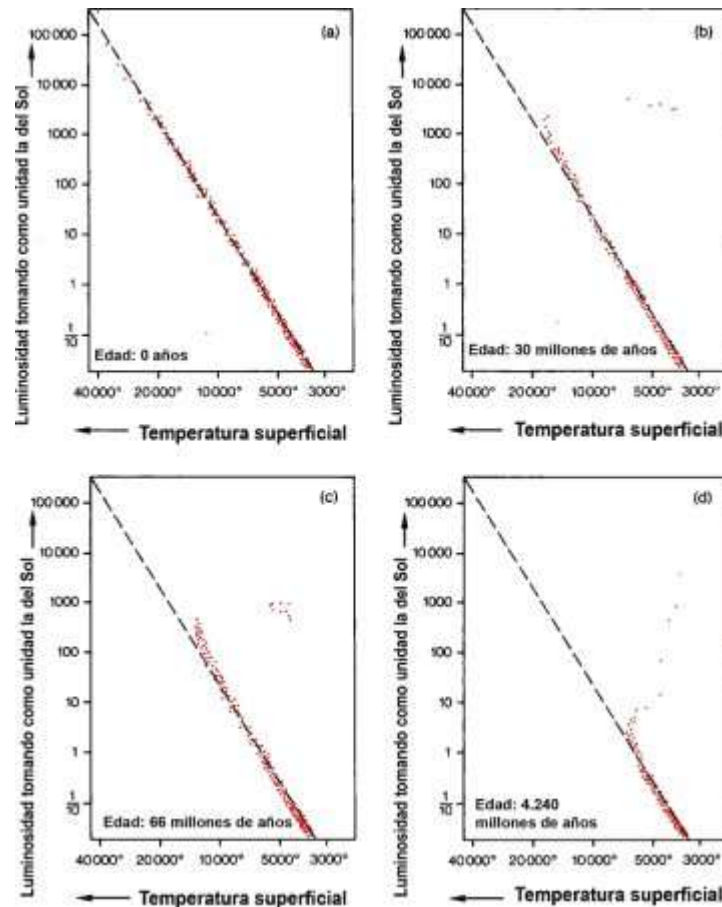
Figura 6-3. Cuatro diagramas HR de un cúmulo estelar imaginario en distintas edades. Cada punto corresponde a una estrella de determinada masa, que en el transcurso del tiempo se desplaza siguiendo la trayectoria evolutiva calculada por el computador. Está señalada la situación de los puntos representativos en cuatro posiciones temporales.
