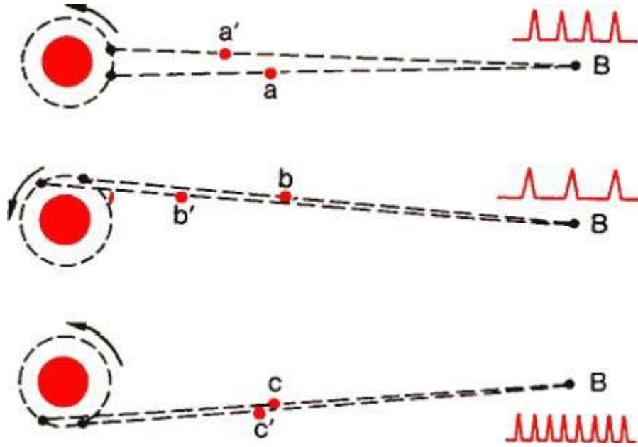
Figura 10-5. Una fuente de rayos X que podría emitir impulsos separados por un segundo gira en una órbita circular alrededor de una estrella representada en la figura como un disco. Un observador B situado a gran distancia del astro mide los intervalos entre dos destellos sucesivos. Arriba: Dos destellos a y a' , en camino hacia el observador. Cuando la fuente emitió a' estaba en un punto de su órbita distinto al de la emisión de a . En el caso aquí representado los trayectos de ambos destellos son de igual longitud. El observador los capta con una separación de un segundo. Centro: Los destellos b y b' emitidos cada segundo han de recorrer ahora trayectos de distinta longitud. El destello b' emitido en segundo lugar ha de cubrir una distancia más larga. El observador recibe ambos destellos con un intervalo de separación superior a un segundo. Abajo: El destello c emitido en segundo lugar recorre el trayecto menor; el observador capta los destellos más juntos.
