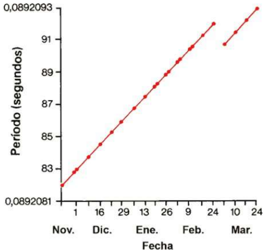
Figura 8-11. Salto periódico de un pulsar. El período del pulsar, que crece lentamente, se acorta de repente (arriba a la derecha) y luego continúa su crecimiento.
