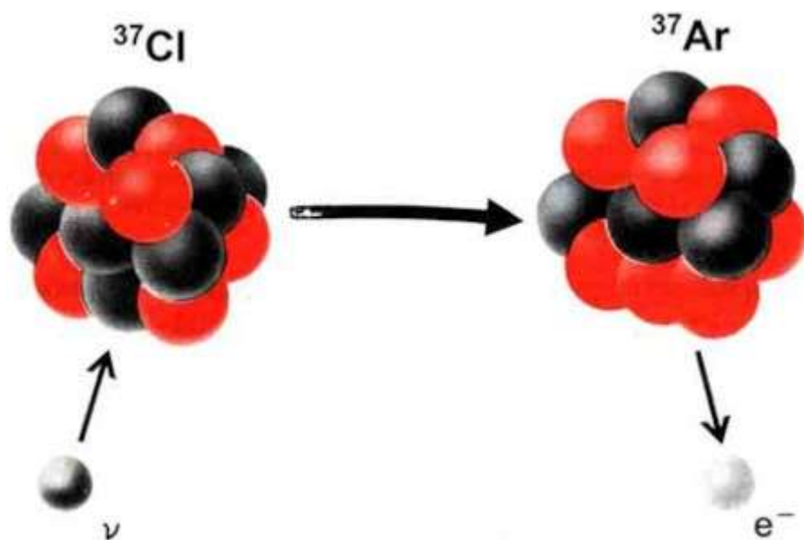
Figura 5-5. Un neutrino puede transformar un átomo de cloro en un átomo de argón. Se libera entonces un electrón.
