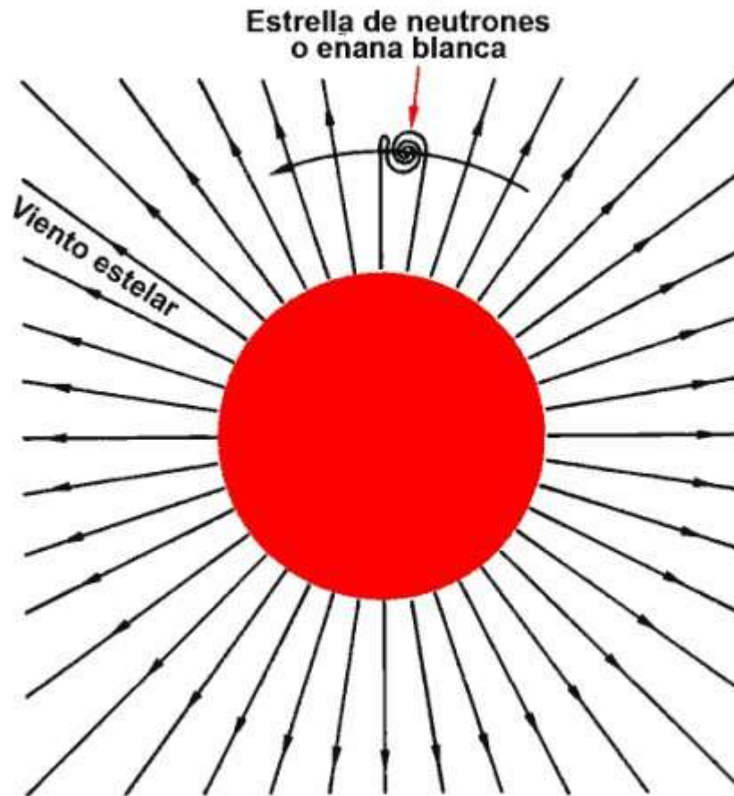
Figura 10-9. Una posible causa de la emisión de rayos X en un sistema estelar doble. Una estrella (en el centro del dibujo) proyecta viento estelar al espacio. Las líneas con flecha que parten de la estrella principal indican la dirección del flujo. Una estrella de neutrones o enana blanca que gira alrededor de la estrella principal, recoge una parte de las masas gaseosas que fluyen por el espacio y las obliga a precipitarse con mayor velocidad sobre su superficie. Al chocar el gas contra la superficie, la materia se calienta hasta emitir rayos X.
