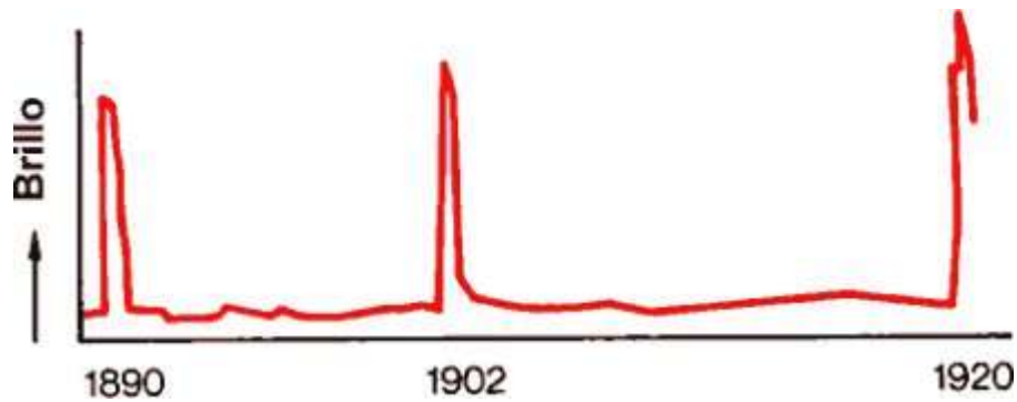
Figura 9-9. Las explosiones de la nova T Pyxidis se repiten a intervalos regulares. Se observaron explosiones en los años 1890., 1902, 1920, 1944 y 1966.
