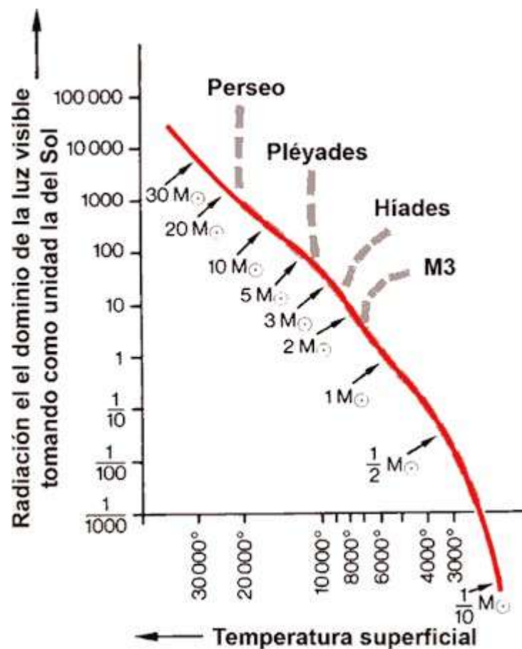
Figura 2-10. Desviación de varios cúmulos estelares con relación a la secuencia principal (según Allen Sandage). Las líneas de trazo grueso indican la situación de las estrellas de varios cúmulos estelares. Un cúmulo de Perseo tiene la secuencia principal de mayor desarrollo
