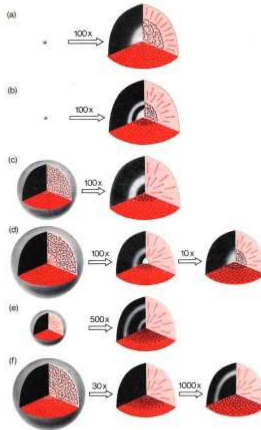
Figura 6-1. Estructura interna de una estrella de siete masas solares en épocas distintas de su evolución. La estrella está representada a la izquierda siempre a la misma escala. Su interior aparece ampliado a la derecha. En fases posteriores de la evolución ha sido preciso ampliar el doble la zona interior para hacerla visible. Los símbolos son los mismos que los de las figuras 4-2 y 5-2. Después de encenderse el helio se forma carbono, representado por circulitos en negro, (a) Modelo de la primitiva secuencia principal con región central convectiva, (b) La estrella 26 millones de años más tarde. Su diámetro no ha cambiado mucho, pero en la región central la combustión central empieza ya a convertirse en combustión pelicular, como puede observarse en el sector superior izquierdo, (c) Pasados 26,5 millones
