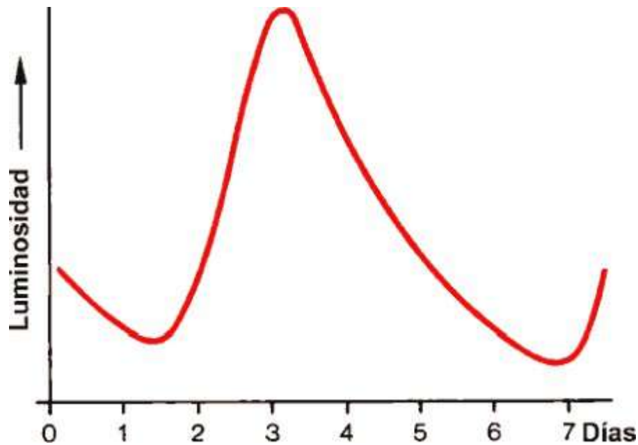
Figura 6-4. Curva de luminosidad de la estrella delta Cephei. La luminosidad de la estrella sube hasta su máximo con un ritmo periódico de 5,4 días, debilitándose luego de nuevo. La trayectoria evolutiva calculada de la estrella de siete masas.
