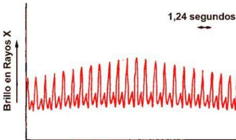
Figura 10-3. Destellos de rayos X de la fuente que Uhuru descubrió en Hércules.
