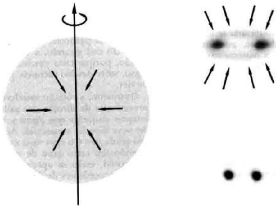
Figura 13-2. Una nube interestelar en rotación se contrae. En el dibujo superior está indicado el eje de rotación. Al principio el gas cae uniformemente hacia el centro desde todas las direcciones, como señalan las flechas rectas. Más tarde (derecha) se forma un disco de rotación sobre el cual cae el gas procedente principalmente de la
