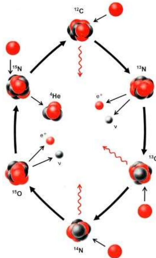
Figura 3-2. Transformación del carbono en helio según el ciclo del carbono. La representación es la misma que la de la figura 3-1. Las flechas onduladas indican que un átomo emite radiación; los positrones están señalados por e^+ y los neutrinos por \nu .
