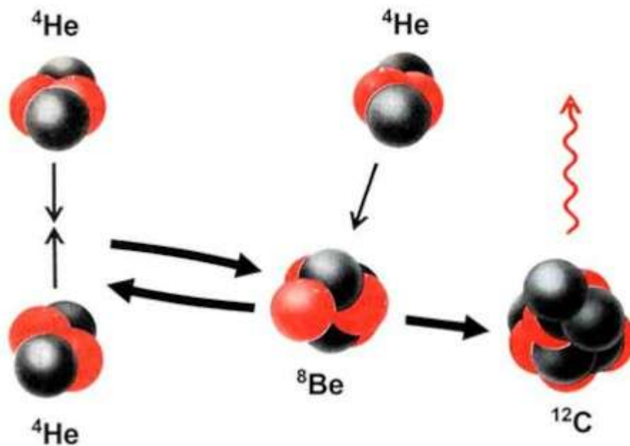
Figura 3-4. Fusión del helio y formación del carbono. Dos núcleos de helio se fusionan formando un núcleo de berilio muy radiactivo que rápidamente se transforma de nuevo en los dos núcleos originales de helio. Pero si durante su corta vida choca con él otro núcleo de helio,
