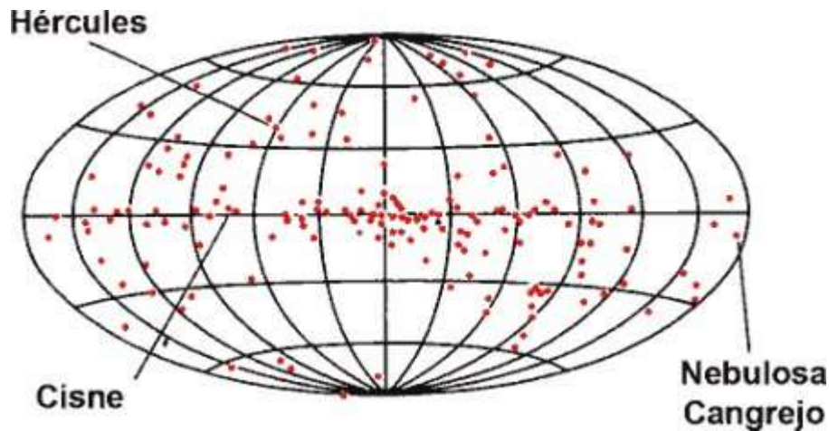
Figura 10-2. Distribución en el cielo de las fuentes de rayos X descubiertas por Uhuru. La red de coordenadas angulares, como la de la figura 8-4, se ha escogido de modo que la esfera celeste quede representada sobre una superficie ovalada. La Vía Láctea se extiende a lo largo de la recta central. En el centro del óvalo miramos exactamente hacia el centro del disco de la Vía Láctea. La mayoría de fuentes de rayos X están situadas en el cielo cerca de la Vía Láctea, especialmente en las proximidades de su centro. Se han señalado algunas fuentes citadas en el texto.
