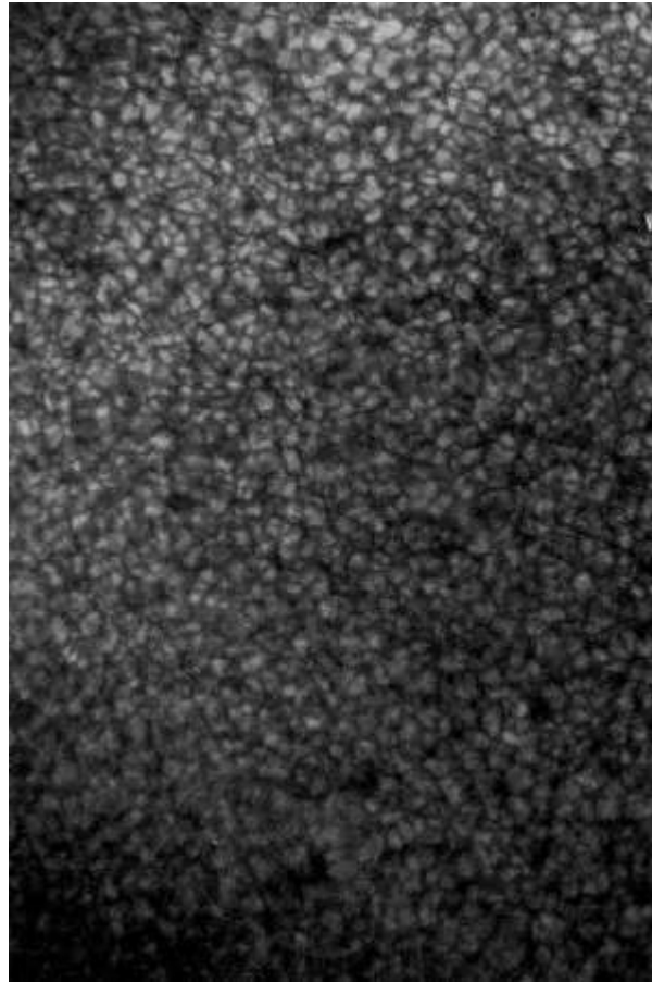
Figura 4-1. Granulación de la superficie solar. En las capas exteriores del Sol la energía procedente del interior se transporta por convección, mediante la subida hasta la superficie solar de globos gaseosos calientes y más brillantes, mientras que se hunden hacia dentro masas gaseosas más frías (más oscuras en la fotografía). Un intervalo igual al diámetro de la Tierra ocuparía en la fotografía una longitud de 14 mm. (Fotografía: D. Soltau con el reflector de vacío de 40 cm del Kiepenheuer-Institut für Sonnenphysik [Friburgo] en Izana [Tenerife].)
