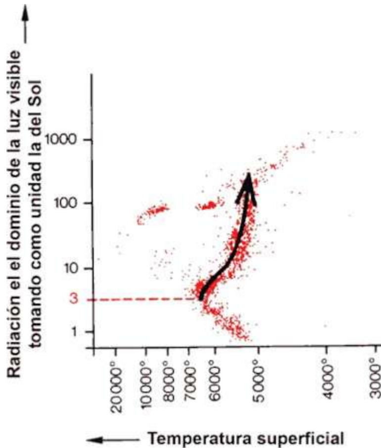
Figura 5-4. Diagrama HR de un cúmulo estelar ya reproducido en la figura 2-9, pero ahora con una trayectoria evolutiva que indica cómo se desplazan las estrellas de la secuencia principal hacia el dominio de las gigantes rojas. La trayectoria evolutiva aquí representada no es comparable cuantitativamente con la trayectoria dada en la figura 5-1 para el Sol por los siguientes motivos: porque las estrellas que han abandonado la secuencia principal tienen una masa algo distinta (las estrellas de masa solar de este cúmulo todavía están en la secuencia principal), porque las estrellas del cúmulo globular tienen una composición algo distinta y porque la radiación total y la radiación en el intervalo visible son distintas. Sin embargo, se observa cualitativamente que las estrellas de este cúmulo globular
