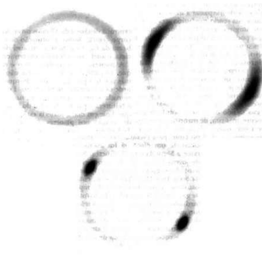
Figura 13-3. La concentración anular de materia formada en la figura 13-2 aparece aquí vista desde arriba, y ampliada tres veces en relación al dibujo inferior de la figura 13-2. Al cabo de unos centenares de miles de años se descompone en dos condensaciones que pueden formar una estrella cada una, las cuales seguirán luego girando una alrededor de otra en un sistema estelar doble.
