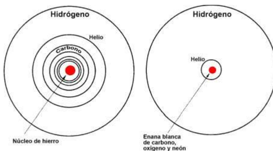
Figura 11-1. Posibles fases preparatorias de una explosión de
