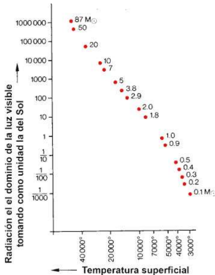
Figura 4-3. Una serie de modelos estelares de distinta masa (formados todos por la misma mezcla química rica en hidrógeno) traza en el diagrama HR una secuencia principal con todas las propiedades de la secuencia principal observada. Las masas de cada modelo están expresadas en unidades de masa solar ( M_{\odot} ). Puede observarse que la radiación de las estrellas de la secuencia principal
