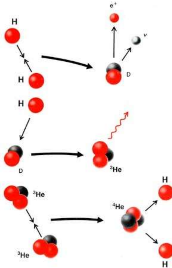
Figura 3-3. Cadena protón-protón. La representación es la misma que la de la figura 3-2. De nuevo el hidrógeno se transforma en helio. En el dibujo superior chocan entre sí dos núcleos de hidrógeno y forman un núcleo de deuterio. En el central se unen un núcleo de deuterio y otro de hidrógeno para formar un isótopo del helio. Debajo se fusionan dos núcleos de este isótopo formando un helio normal de número másico 4.
