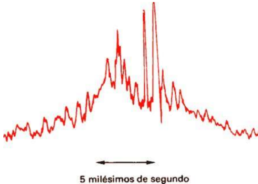
Figura 8-2. Impulso aislado registrado con mayor resolución temporal, Las señales del pulsar presentan una estructura fina complicada.
