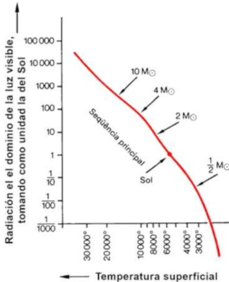
Figura 2-3. Diagrama HR con la secuencia principal (indicada esquemáticamente con la línea curva). En cada punto de la secuencia principal sólo hay estrellas de una masa determinada. (El astrónomo utiliza a menudo la masa del Sol como unidad de masa, y la respuesta por M_{\odot} .)
