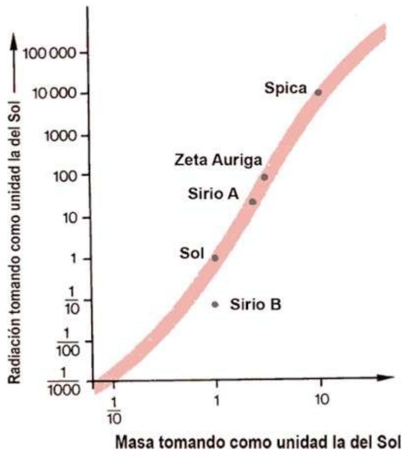
Figura 2-4. Si representamos en un diagrama la luminosidad creciendo hacia arriba y la masa estelar creciendo hacia la derecha, las estrellas de la secuencia principal quedan situadas sobre una estrecha banda: cuanto mayor es la masa de una estrella, mayor es su luminosidad. Esta es la relación masa-luminosidad. Pero sólo es válida para estrellas de la secuencia principal. La acompañante de Sirio, Sirio B, incluida en el diagrama emite menos energía que una estrella de la secuencia principal de igual masa. Sirio B no cumple la relación.
