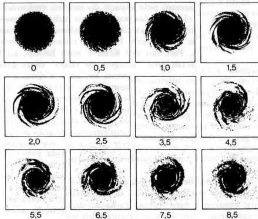
Figura 12-6. Modelo simplificado de computador del movimiento de las estrellas en nuestra galaxia. Alrededor del centro de un disco plano, que aquí vemos desde arriba, se mueven 200.000 estrellas. Los números de cada recuadro indican el tiempo transcurrido desde la distribución inicial del primer recuadro. La unidad utilizada es el tiempo medio necesario para una revolución. Por tanto, el tiempo transcurrido entre el primer y el tercer recuadro es exactamente el necesario para que la Vía Láctea dé una vuelta sobre sí misma. Pronto se forma una estructura espiral. En el brazo espiral superior de los dibujos correspondientes a las épocas 4,5 y 5,5 puede comprobarse que las espirales constituyen lugares de paso, es decir, que en cada momento están formadas por estrellas distintas. Puede verse también que el brazo del recuadro siguiente es un producto del anterior. Entre los dos recuadros el brazo ha girado poco. En cambio,
