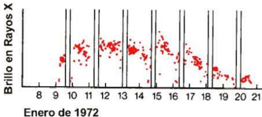
Figura 10-6. Comportamiento de la fuente Hércules X-1 en un intervalo prolongado de tiempo. Los puntos indican la intensidad de los destellos de rayos X medidos por Uhuru. Las líneas dobles verticales están dibujadas a intervalos de 1,70017 días. Indican el intervalo de cinco horas durante el cual desaparecen los destellos al ocultarse la fuente detrás del astro alrededor del cual está girando. Los impulsos empezaron a captarse el 9 de enero y después del 21 desaparecieron. La desaparición responde al ciclo de treinta y cinco días de la fuente de Hércules explicado en el texto.
