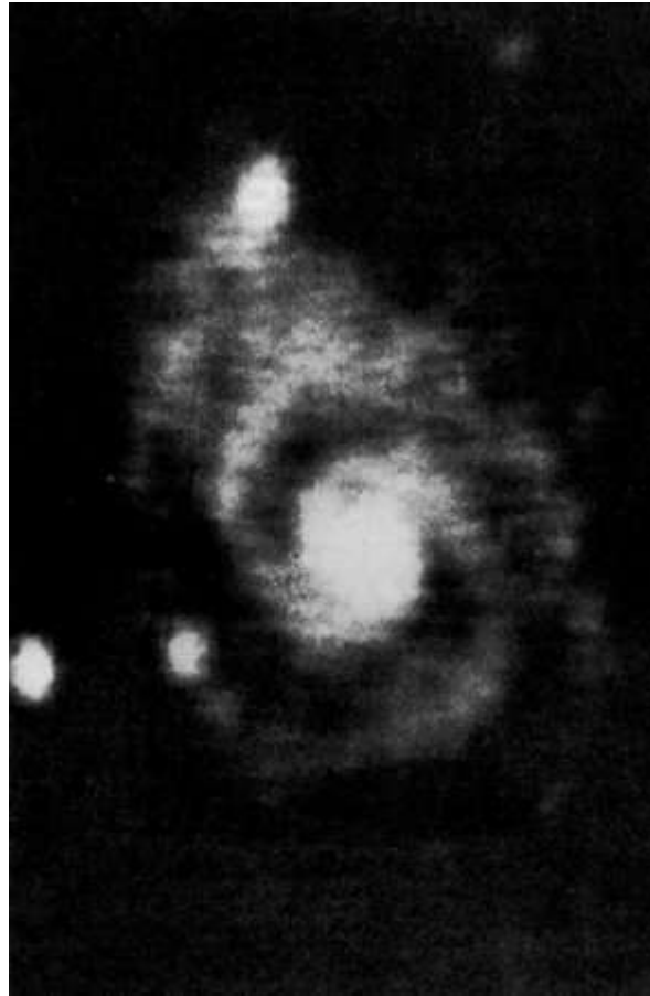
Figura 12-7. Imagen de radio de la galaxia de la figura 0-4. Esta imagen trazada por computador nos muestra la galaxia tal como aparecería ante nuestros ojos si éstos fueran sensibles a las emisiones de radio de 21 cm de longitud de onda y pudieran "ver" tan bien como el gran radiotelescopio de Westerbork, en Holanda. La radiación de esta longitud de onda llega principalmente de zonas donde el gas interestelar tiene una densidad elevada. La imagen de radio nos indica, por tanto, que el gas de esta galaxia tiene casi la misma estructura espiral que la distribución de estrellas jóvenes. (Fotografía: Sterrewacht Leiden.)
