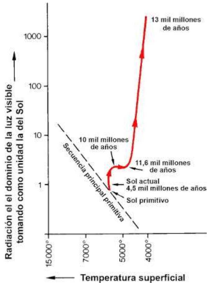
Figura 5-1. Trayectoria evolutiva del Sol en el diagrama HR. La evolución parte del Sol primitivo, pasa por el Sol actual, se separa de la secuencia principal primitiva y se dirige al dominio de las gigantes rojas. Las indicaciones de edad señalan el tiempo transcurrido desde el momento de encenderse el hidrógeno en el Sol primitivo.
