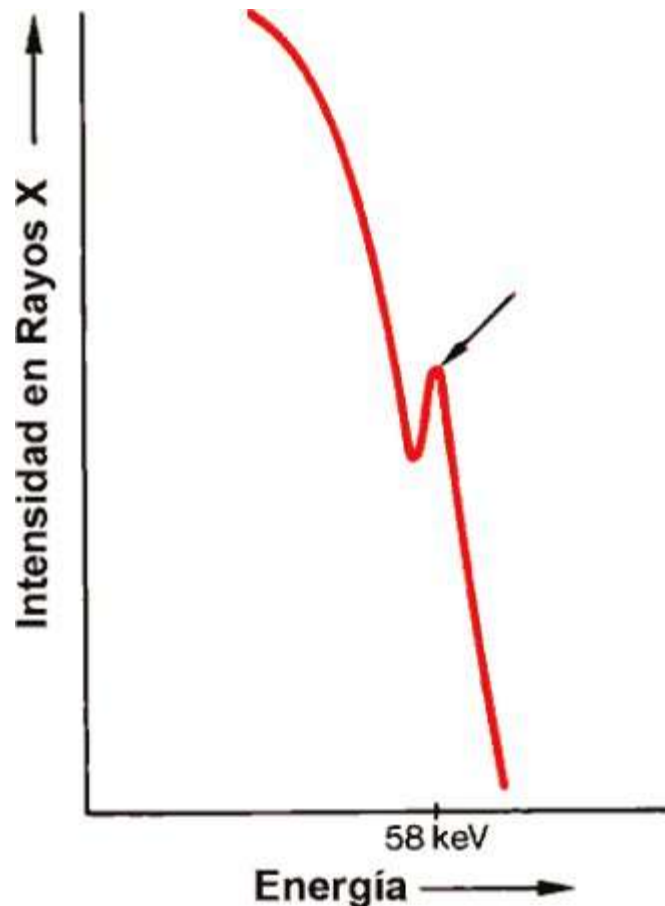
Figura 10-12. Emisión de rayos X de la fuente Hércules X-1 en el dominio de las altas energías. Lo normal sería que la radiación de la fuente disminuyera hasta las altas energías. Sin embargo, aparece una irregularidad en los 58 kiloelectronvoltios, en forma de pico (señalado por la flecha). Cuando las energías son tan altas es difícil medir la radiación de la fuente; no es pues seguro que la distribución real de la energía siga exactamente la línea dibujada.
