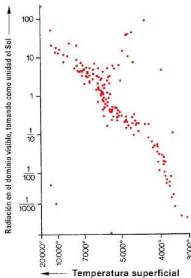
Figura 2-2. Estrellas vecinas del Sol en el diagrama MR. La mayoría de estas estrellas tienen temperaturas superficiales y luminosidades tales que sus puntos representativos caen sobre una banda del diagrama que va de la parte superior izquierda a la parte inferior
