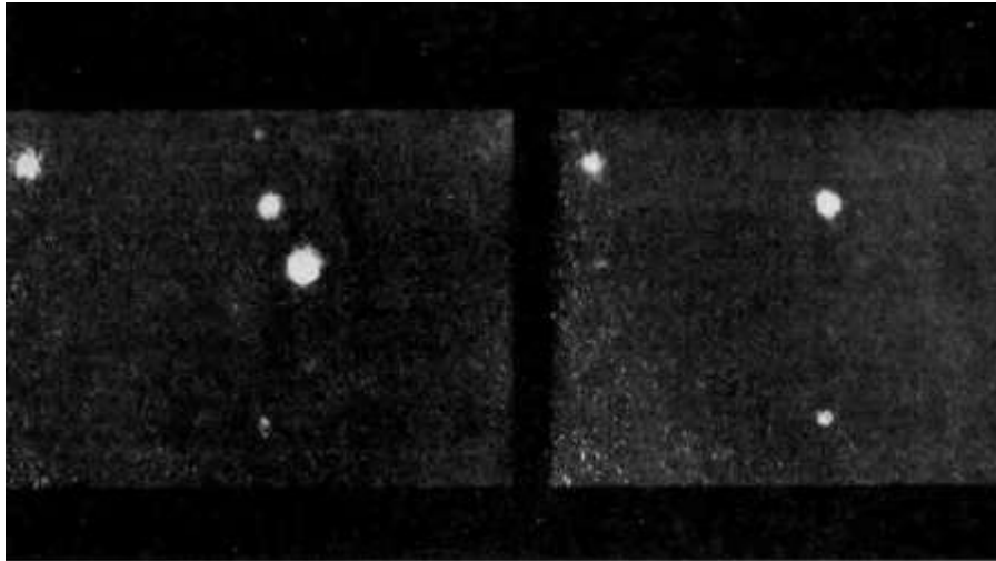
Figura 8-8. Dos imágenes construidas con el método de las dos pantallas de televisión (véase fig. 8-6) permiten descubrir que una de las estrellas de la figura 8-5 emite su luz siguiendo el ritmo del pulsar del Cangrejo. La estrella está señalada en la figura 8-5 con dos marcas blancas en el borde derecho e inferior. Comparando la figura 8-5 con la figura 7-6 puede encontrarse fácilmente en la fotografía en color el pulsar del Cangrejo, que allí no se distingue en nada de las demás estrellas. (Fotografía: Observatorio Lick.)
