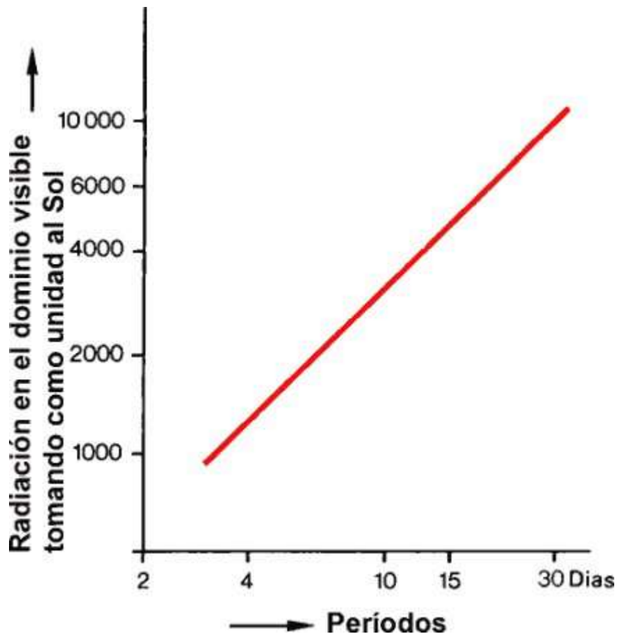
Figura B-2. Relación período-luminosidad de las estrellas cefeidas. A cada período de estas estrellas corresponde una luminosidad concreta. Los períodos pueden determinarse fácilmente; por tanto, puede deducirse inmediatamente la luminosidad media correspondiente a este período. Esta luminosidad, comparada con el brillo aparente de la estrella en el cielo, nos da su distancia.
