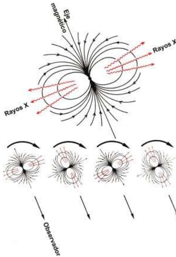
Figura 10-11. Origen de los destellos de rayos X. Cuando cae materia sobre una estrella compacta, el choque genera rayos X (parte superior de la figura). Si la estrella posee un campo magnético de forma semejante al campo terrestre, es decir, cuyas líneas de campo tienen la forma de las líneas ovaladas trazadas en la figura, el gas sólo puede precipitarse sobre la estrella compacta, representada por una bolita, siguiendo las líneas de campo que apuntan en la dirección de las flechas a los dos polos. La materia que cae en las proximidades del eje magnético forma dos “tapones” opacos a los rayos X. Por tanto, la radiación generada sólo puede escapar al espacio lateralmente (flechas onduladas). Si gira todo el astro, puede suceder que un observador lejano sólo capte los rayos X durante un breve
