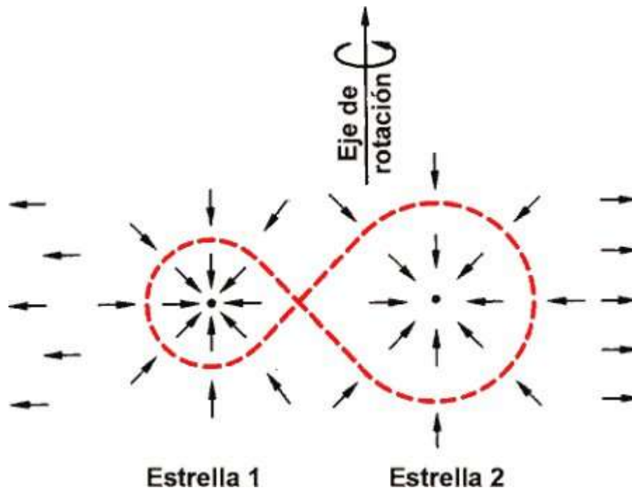
Figura 9-1. Fuerzas presentes en un sistema estelar doble. Las dos estrellas están bufadas como puntos. Las flechas indican en qué dirección actúa la fuerza sobre un átomo de gas situado en cada punto. En las cercanías de cada estrella domina su gravedad, y las flechas señalan o bien hacia la estrella 1 o bien hacia la estrella 2. En la línea de unión de las dos estrellas hay un punto donde se equilibran exactamente las fuerzas de atracción de las estrellas. Las estrellas giran una alrededor de la otra (el eje del movimiento giratorio y la dirección de giro están indicadas en la mitad superior
