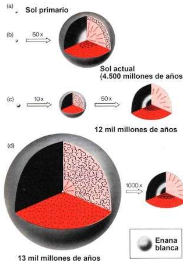
Figura 5-2. Estructura interior de los modelos solares en distintas fases de evolución. La representación es la misma que la de la figura 4-2. Ahora, contrariamente a la figura indicada, tenemos regiones en las que el helio se ha enriquecido; unos circulitos señalan allí la presencia del helio recién creado, que todavía está mezclado parcialmente con la materia original rica en hidrógeno, indicada por puntos. Más tarde en la región central sólo queda helio. A la izquierda están dibujados los modelos a la misma escala (pero no a una escala igual a la de los dibujos de la izquierda de la fig. 4-2) y a la derecha
