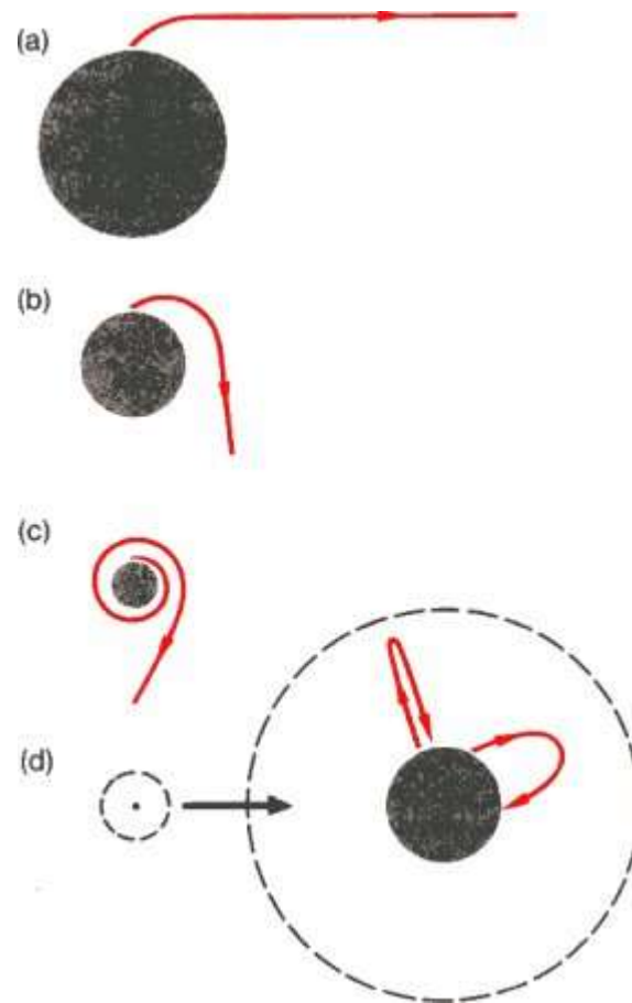
Figura 11-3. Desviación de la luz en las proximidades de una estrella de neutrones en colapso, (a) La luz emitida por la estrella se curva cerca de su superficie, (b) Cuanto más pequeño es el radio de la estrella, más fuerte es la curvatura, de modo que en (c) un rayo de luz emitido oblicuamente por la superficie ha de luchar contra la gravedad y recorrer varias vueltas de espiral antes de poder escapar de la estrella, (d) La estrella es ahora más pequeña que su radio de Schwarzschild. Todos los rayos luminosos que emite su superficie se curvan y caen de nuevo sobre la estrella. El dibujo de la izquierda en (d) está ampliado el doble en relación a (c). La estrella es ahora muy pequeña en comparación con las fases anteriores y en el dibujo de la derecha aparece más ampliada todavía. Los círculos discontinuos
