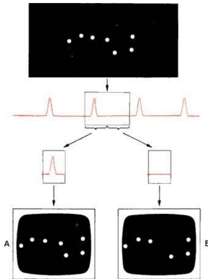
Figura 8-6. Principio que permite reconocer si una estrella emite su luz de modo uniforme o por impulsos. Arriba vemos el grupo estelar sin cambios especiales. Debajo están los destellos periódicos de luz de una de las estrellas. La imagen captada por una cámara de televisión se transmite siguiendo el ritmo del período estelar a dos pantallas de televisión A y B. La pantalla A recibe siempre la imagen con impulso, la pantalla B recibe la imagen cuando la estrella no emite impulso. Comparando las dos imágenes (debajo) puede reconocerse la estrella que emite su luz con pulsaciones. (El método aparece aplicado aquí a una estrella de la Osa Mayor. Esta estrella no es en realidad un pulsar, es una estrella totalmente inofensiva que nos envía su luz de
