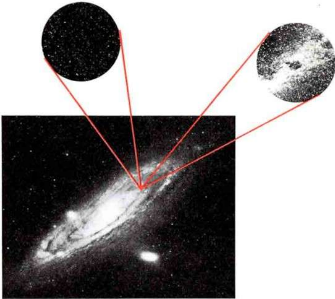
Figura 0-2. El ejemplo de la galaxia de Andr meda nos permite entender el origen de la banda luminosa de la V a L ctea. Si un observador, desde su planeta nativo situado en el disco gal ctico, mira hacia fuera del plano del disco ver  m s o menos la imagen de la izquierda: en su campo de visi n aparece un n mero relativamente reducido de estrellas. Si mira en una direcci n que coincida con el plano del disco, ver  la multitud de estrellas del disco formando una banda luminosa que cruza el cielo, como muestra la imagen de la parte superior derecha.
