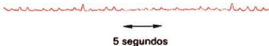
Figura 8-1. Señales del primer pulsar descubierto sobre la cinta registradora. Los impulsos individuales no tienen la misma forma, pero se suceden a distancias regulares con gran precisión
