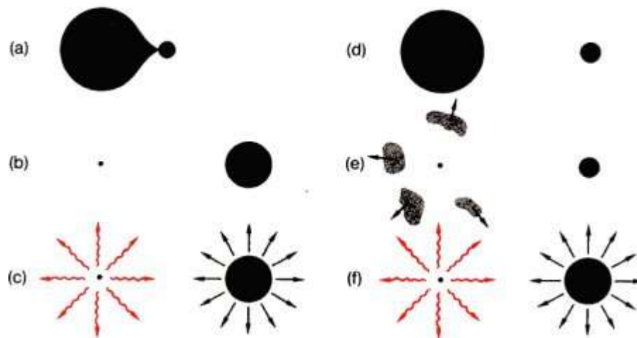
Figura 10-10. Dos posibles historias evolutivas de sistemas estelares que pueden producir una fuente de rayos X. izquierda: dos estrellas de la secuencia principal y de masas distintas giran una alrededor de la otra a poca distancia. La de mayor masa presenta primero los síntomas de agotamiento, y podría convertirse en una gigante roja. Pero sus capas exteriores se introducen en el dominio gravitatorio de la acompañante, y ésta le absorbe tanta masa (a), que sólo le queda el núcleo en forma de enana blanca, tal como está representada en (b) de la figura 9-6. Si la estrella de la derecha que se ha convertido ahora en la de mayor masa genera en el curso de su evolución un viento estelar, una parte del gas proyectado cae sobre la enana blanca que puede emitir rayos X (flechas onduladas), como indica la
