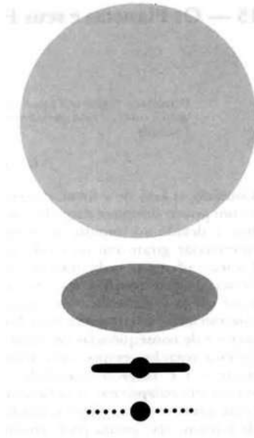
Figura 13-1. Esquema de la formación de nuestro sistema planetario.
