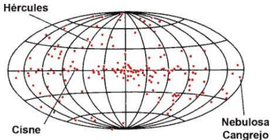
Figura 8-4. Distribución de 300 pulsares en el cielo. La red de coordenadas angulares está elegida de modo que toda la esfera celeste quede representada en la superficie oval de la red. La Vía Láctea se extiende a lo largo de la línea media horizontal. El centro del disco de la Vía Láctea está situado en el medio. La mayoría de los pulsares están situados cerca de la Vía Láctea.
