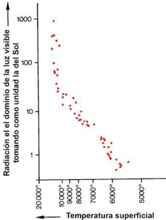
Figura 2-7. Diagrama HR del cúmulo estelar de las Pléyades. Sólo están representadas las estrellas más brillantes. El diagrama muestra una secuencia principal muy marcada. Pero hacia arriba, cuando la luminosidad visual es más de mil veces la del Sol, las estrellas del diagrama se desvían algo hacia la derecha de la secuencia principal.
