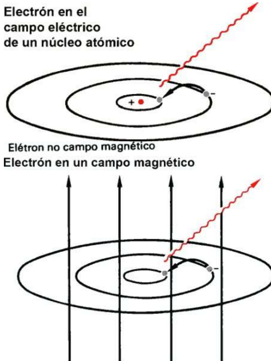
Figura 10-13. Arriba: Un átomo emite radiación (flecha ondulada) cuando un electrón salta de una órbita circular exterior del núcleo atómico positivo a una interior. La radiación tiene una energía muy determinada, característica del átomo y de esta transición concreta. Debajo: En un campo magnético intenso (representado por las flechas rectas y verticales) los electrones sólo pueden moverse en pequeñas órbitas circulares, de modo semejante a los electrones que giran
