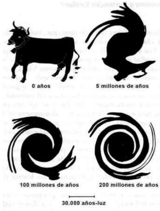
Figura 12-5. La Vía Láctea no gira rígidamente. Por ello al cabo de 100 millones de años una estructura inicial cualquiera habrá dado lugar a una forma espiral. Por desgracia, las espirales de la galaxia no pueden explicarse de este modo.
