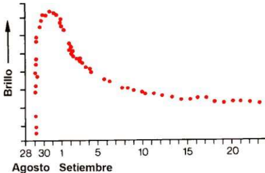
Figura 9-7. Explosión luminosa de la nova del 29 de agosto de 1975 en la constelación del Cisne. Los puntos representan observaciones
