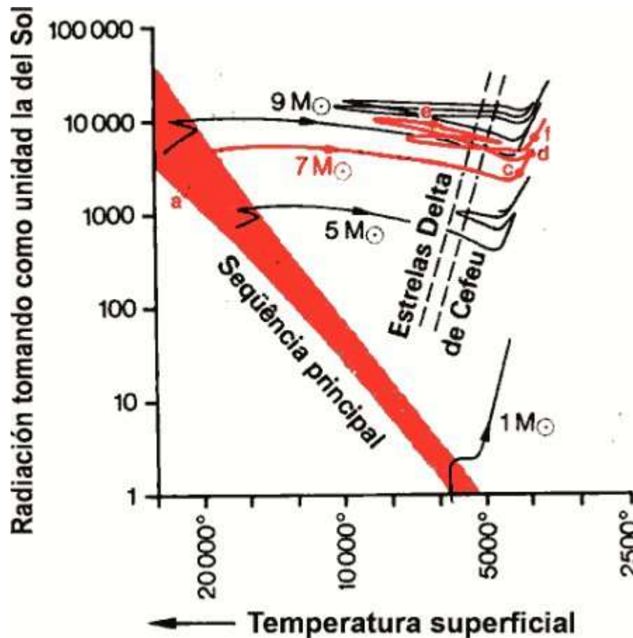
Figura 6-2. Trayectoria evolutiva de estrellas de distinta masa. Los números que acompañan a las trayectorias indican las respectivas masas en unidades de masa solar. La trayectoria de una masa solar, que vimos ya en la figura 5-1 lleva a la región de las gigantes rojas, pero las trayectorias evolutivas de estrellas de mayor masa llevan a estrellas rojas todavía más grandes del dominio de las supergigantes. Las letras de la trayectoria evolutiva de la estrella (a-f) de siete masas solares, se refieren a los modelos representados en los dibujos parciales de la figura 6-1. Las dos rectas paralelas de trazos limitan la banda donde se encuentran las estrellas cefeidas.
