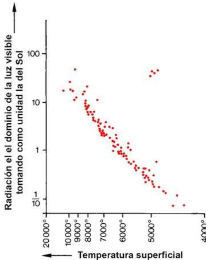
Figura 2-8. Diagrama HR del cúmulo estelar de las Híades. En las Pléyades (véase fig. 2-7) la radiación de las estrellas de la secuencia principal alcanzaba un valor mil veces superior al del Sol; en cambio, la secuencia principal de las Híades se acaba ya por debajo de cien veces la radiación solar. Faltan las estrellas más brillantes de la secuencia principal. En cambio, en el diagrama HR de este cúmulo estelar aparece un grupo de gigantes rojas.
