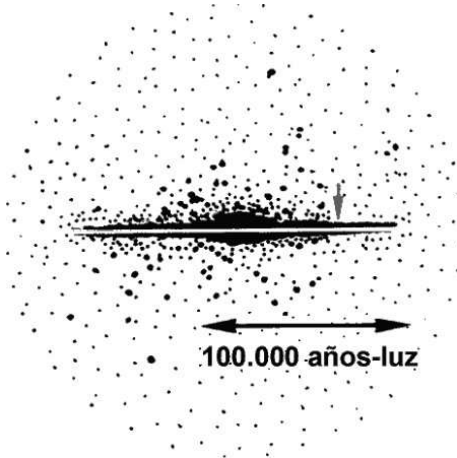
Figura 12-3. Estructura esquemática de la galaxia Vía Láctea. La mayoría de estrellas están situadas en un disco plano que vemos de lado en el dibujo. La flecha señala la situación del Sol, y la banda central clara representa las masas absorbentes de polvo. Los cúmulos globulares (puntos gruesos) y las estrellas muy viejas (dibujadas en la figura como puntitos) constituyen el halo de la Vía Láctea. Las estrellas del halo se formaron hace mucho tiempo. Actualmente sólo nacen estrellas en las proximidades inmediatas del plano central recubierto de masas de polvo.
