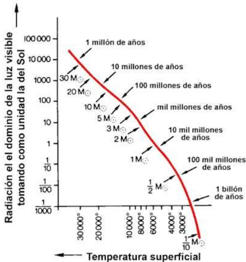
Figura 2-11. Secuencia principal del diagrama HR. A la izquierda las flechas indican la situación que ocupan en la secuencia principal estrellas de masas determinadas (tomando de nuevo como unidad la masa solar M_{\odot} ). La masa determina la reserva de energía a disposición de cada estrella y este dato junto con la luminosidad que corresponde a cada punto de la secuencia principal permite calcular el tiempo durante el cual una estrella situada en un punto concreto puede mantener su luminosidad actual con las reservas de que dispone. Las flechas de la derecha indican los correspondientes intervalos de tiempo. Las estrellas cuya masa es igual a 30 masas solares apenas duran con sus reservas de hidrógeno un millón de años. Las estrellas de media masa solar pueden durar casi cien mil
