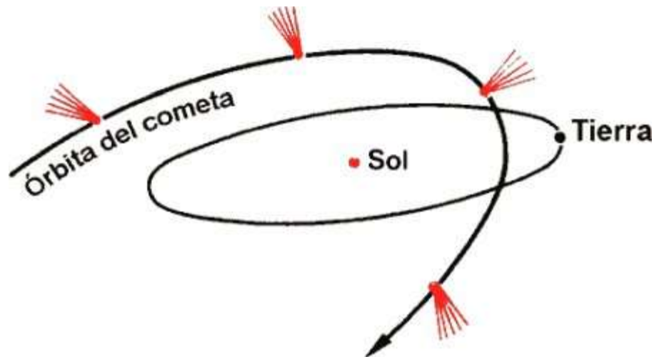
Figura 7-4. El cometa al avanzar por su órbita mantiene siempre la cola gaseosa en dirección opuesta a la del Sol.
