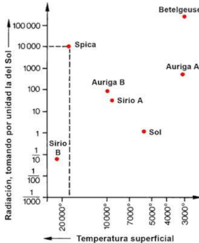
Figura 2-1. Diagrama de Hertzsprung-Russell con algunas estrellas que ya conocemos. Cuando se conoce la temperatura superficial de una estrella se parte de la temperatura correspondiente en la escala horizontal y se sube hacia arriba. Si se conoce también la luminosidad, se parte del valor correspondiente en la escala vertical de radiación y se tira hacia la derecha. La estrella está representada en el punto de intersección de ambas rectas. Dos rectas de trazos que corresponden a la estrella Spica (temperatura superficial, 18.000°; luminosidad, 10.000 luminosidades solares) indican cómo se representa una estrella en el diagrama.
