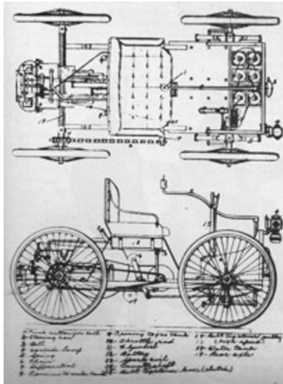
Diseño para el primer Ford.
